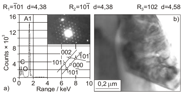
Figure 8. a) X-ray spectrum and diffraction from precipitate, b) Transmission electron micrograph of Al 2 O 3 C precipitate and SADP showing [020] zone axis orientation of Al 2 O 3 C in the inset Slika 8. a) EDX i difrakcija iz precipitata, b) TEM precipitata Al 2 O 3 C i SADP pokazuje [020] zonu orijentacije osi u Al 2 O 3 C u umetku
