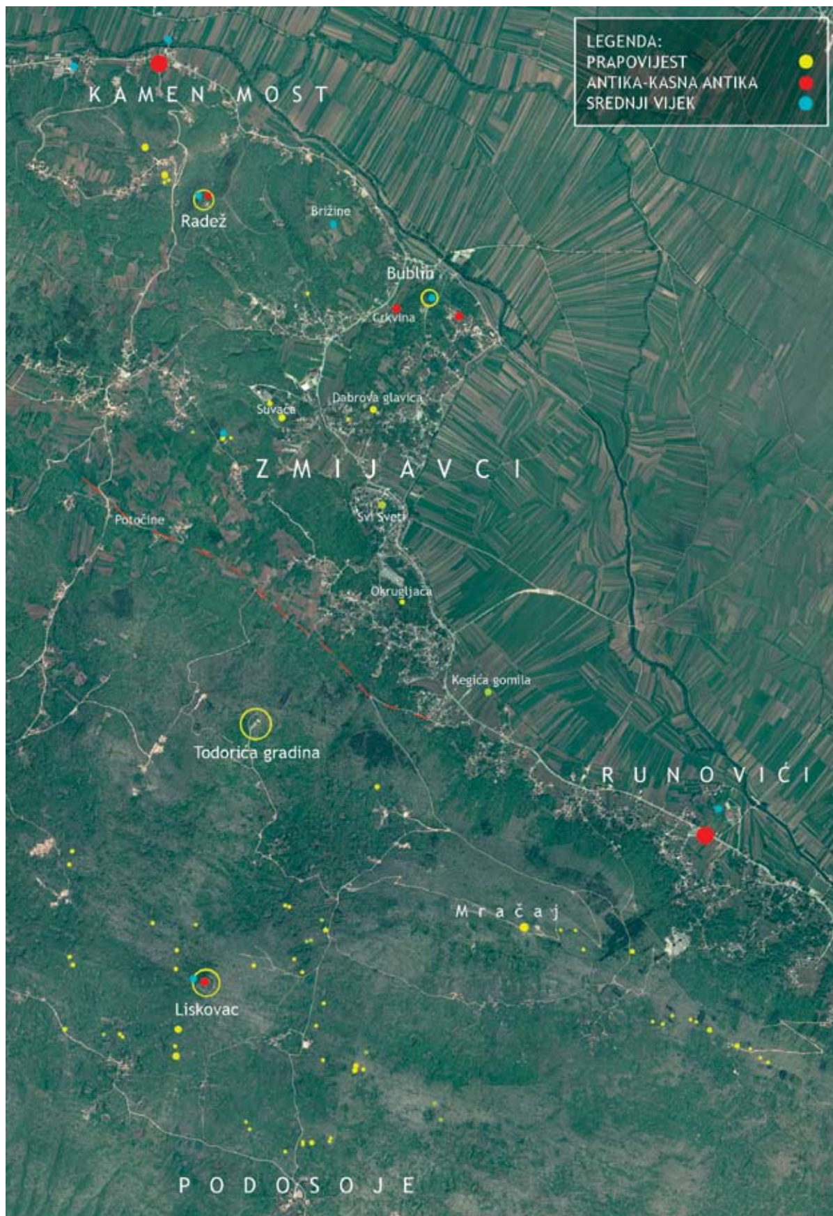
Sl. 3. Zmijavci, arheološki lokaliteti
