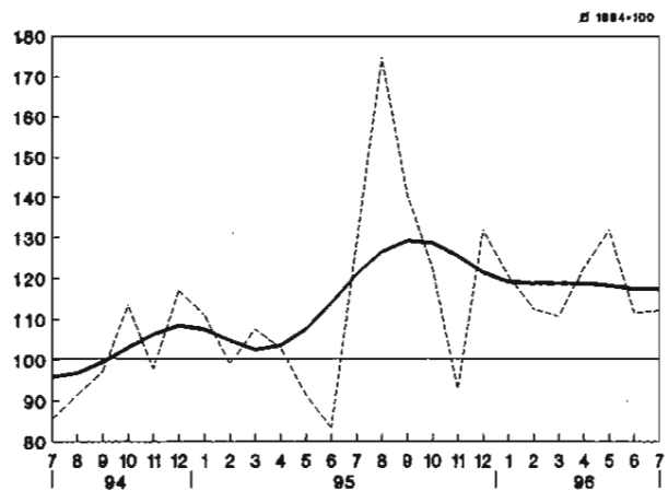
- STROJOGRADNJA -
