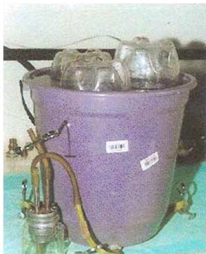
Figura 1. Recipiente confeccionado para o armazenamento de gases produzidos no processo fermentativo "in vitro".
