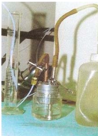
Figura 3. Recipiente de transferência após a injeção de gás no cromatógrafo gasoso pelo acréscimo de água
