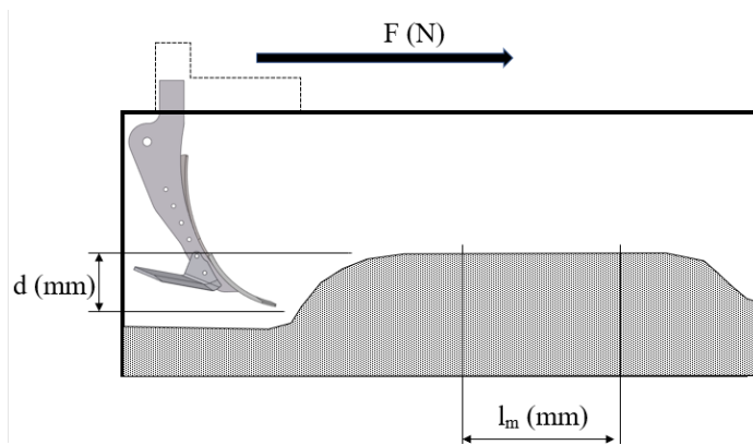
Figure 1. Schema of soil box (Kuře et al., 2020).
