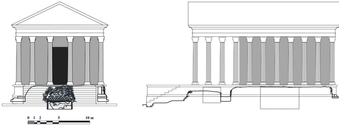
Çizim 3: Akropolis Tapınağı, pseudo-peripteros plana uygun görünüm çizimleri (Baran –Dirlik-Kendirci 2015: Çiz. 4).
