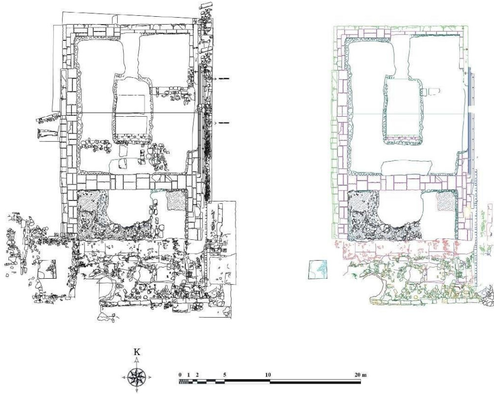
Çizim 1: Tios Akropolis Tapınağı kalıntıları ve planı (Baran-Dirlik-Kendirci 2015: Çiz. 1-2).
