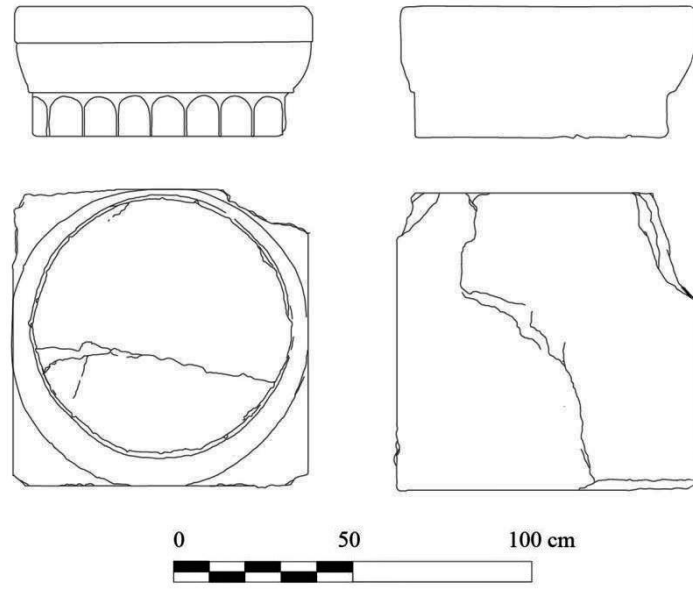
Çizim 5: Akropolis Tapınağı, Dor sütun başlıkları (Baran-Dirlik-Kendirci 2015: Çiz. 7).
