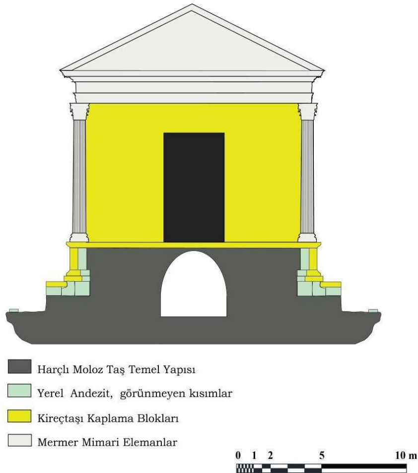
Çizim 4: Akropolis Tapınağında kullanılan taş cinsleri belirtilmiş kesit (Baran-Dirlik-Kendirci 2015: Çiz. 5).
