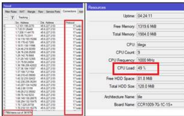
FIGURA 15. Consumo de CPU Ataque UDP-flood. Autores.
