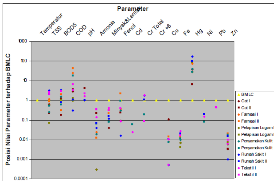
Gambar 2. Perbandingan Baku Mutu Limbah Cair (BMLC) dengan Efluen IPAL pada Pengambilan Sampel (PS) I dan II beberapa Jenis Industri/Kegiatan di Kota Cimahi
