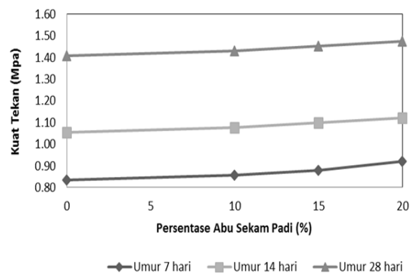
Gambar 3. Hubungan kuat tekan dengan umur beton
