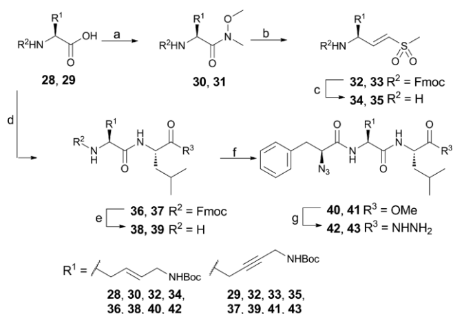
Scheme 2. Synthesis of Lys(4-ene) and Lys(4-yne) vinyl sulfones and peptide hydrazides. Reagents and conditions: a) HCTU [O-(1 H -6-chlorobenzotriazole-1-yl)-1,1,3,3-tetramethyluronium hexafluorophosphate], N,O -dimethyl hydroxylamine; 30 : 100 %, 31 : 85 %; b) 1) \text{LiAlH}_4 , THF; 2) diethyl[(methylsulfonyl)methyl]phosphonate, NaH, THF; 32 : 40 %, 33 : 70 %; c) \text{Et}_2\text{NH} , MeCN; 34 : 70 %, 35 : 47 %; d) H-Leu-OMe, HCTU, DiPEA, \text{CH}_2\text{Cl}_2 ; 36 : 96 %, 37 : 76 %; e) piperidine, DMF; 38 : 94 %, 39 : 100 %; f) \text{N}_3 -Phe-OH, HCTU, DiPEA, \text{CH}_2\text{Cl}_2 ; 40 : 60 %, 41 : 91 %; g) hydrazine monohydrate, MeOH, 100 %.
