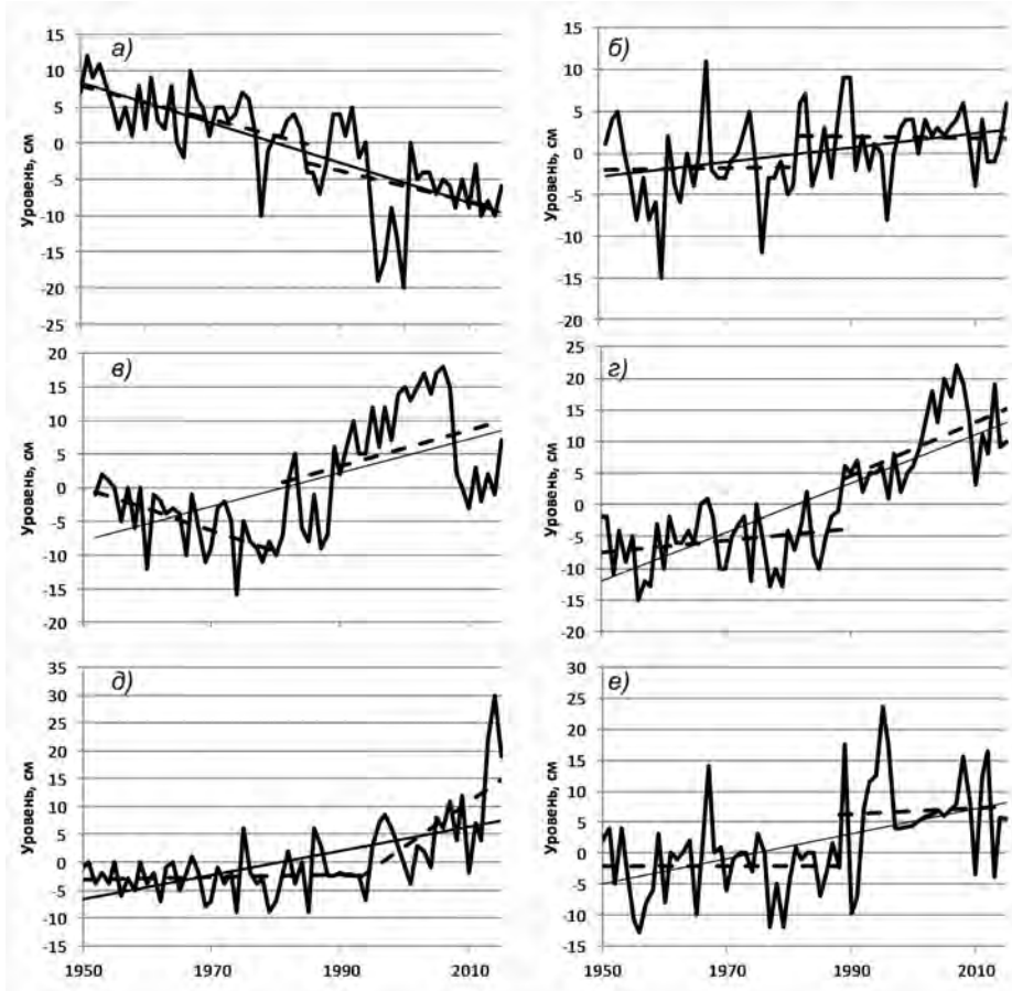
Рис. 2. Аномалии многолетнего хода уровня на станциях: а) — Баренцбург; б) — Олесунн; в) — Мурманск; г) — Амдерма; д) — Усть-Кара; е) — о. Диксон. Прямыми линиями представлены линейные тренды для разных периодов.
