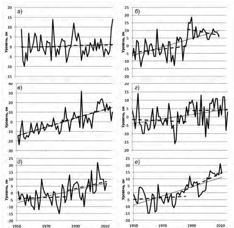
Рис. 3. Аномалии многолетнего хода уровня на станциях: а) — о-ва Известий ЦИК; б) — ГМО им. Е.К. Федорова (бывш. Мыс Челюскина); в) — о. Котельный; г) — пр. Санникова; д) — о-ва Дунай; е) — Певек. Прямыми линиями представлены линейные тренды для разных периодов.
