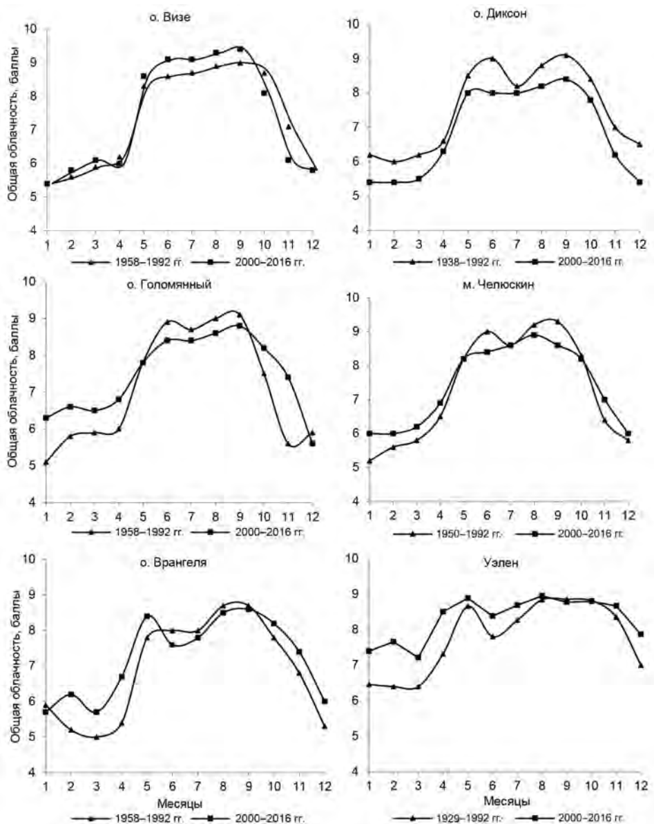
Рис. 1. Сравнение средних значений общей облачности на ряде арктических станций за многолетний период и после 2000 г.
