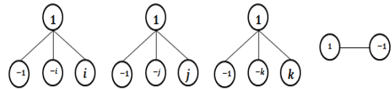
Gambar 3.2.2 Graf koprima dari subgrup quaternion
