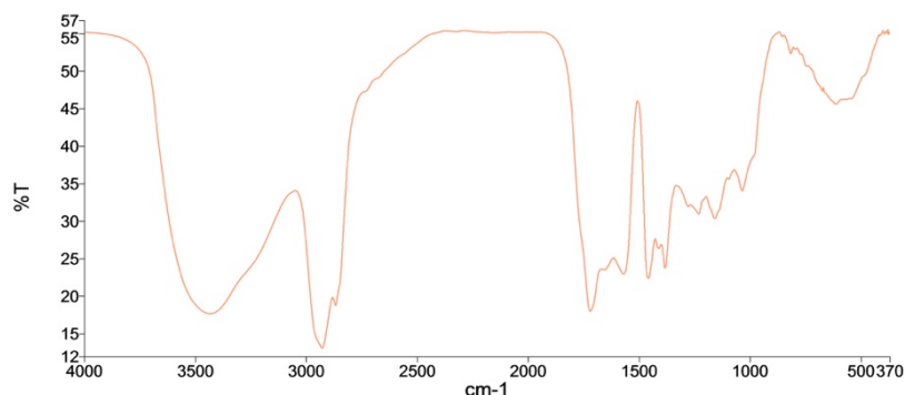
Fig. 5. Espectro FTIR característico del ámbar de La Velilla, presentado en transmisión de infrarrojos.
