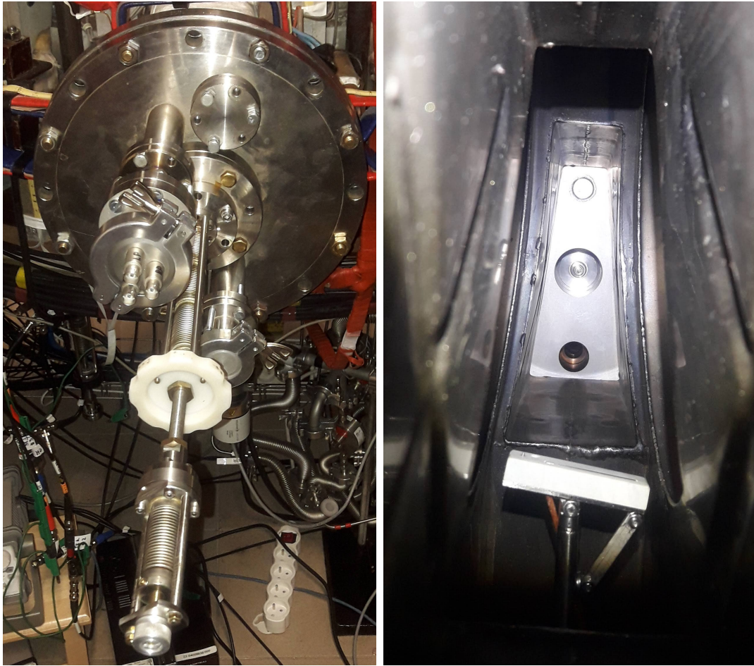
Obr. 2.2: Manipulátor rail sondy instalovaný na LFS tokamaku GOLEM (fotografie nalevo). Hlavice rail sondy uvnitř komory při pohledu z horního portu (fotografie napravo).
