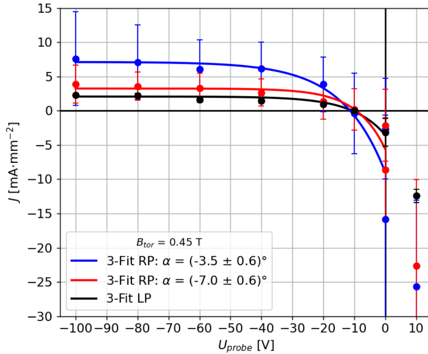
Obr. 3.12: Tři volt-ampérové charakteristiky rail sondy (RP) normované na projekční plochu Rov. 1.36 a složená volt-ampérová charakteristika Langmuirovy sondy (LP) normovaná na plochu Rov. 1.23. Výsledné parametry tříparametrových fitů (3-Fit) jsou uvedeny v tabulce Tab. 3.2.
