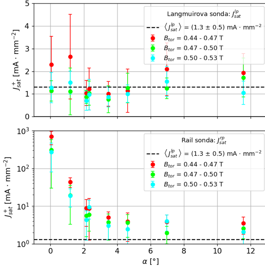
Obr. 3.30: Závislost J_{sat}^+ Langmuirovy (horní část) a rail (dolní část) sondy na úhlu náklonu \alpha pro různé velikosti magnetického toroidálního pole B_{tor} . Černá čárkovaná úsečka představuje střední hodnotu \langle J_{sat}^{lp} \rangle = (1,3 \pm 0,5) \text{ mA} \cdot \text{mm}^{-2} Langmuirovy sondy.
