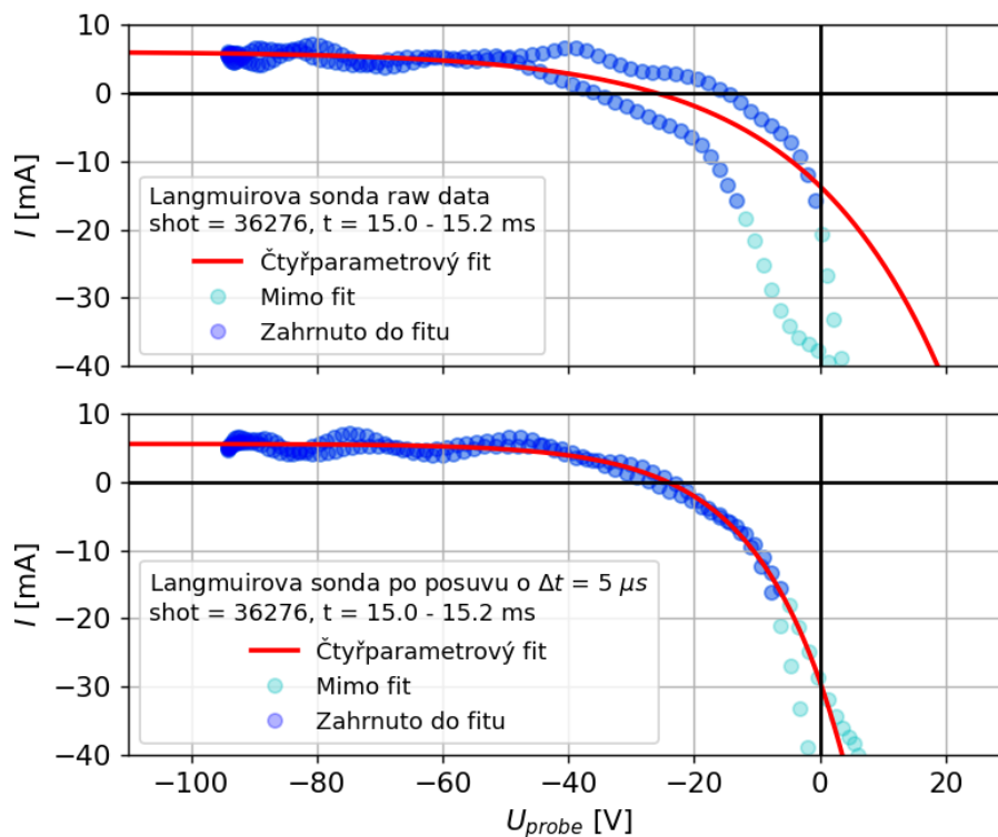
Obr. 3.4: Volt-ampérová charakteristika naměřená Langmuirovou sondou bez úprav a s viditelnou hysterezí (graf nahoře). Po provedení posuvu o 5 \mu s hystereze vymizí (graf dole).
