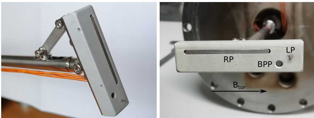
Obr. 2.4: Hlavice rail sondy před instalací na tokamak GOLEM (fotografie nalevo). Odinstalovaná hlavice z tokamaku GOLEM po zhruba 350 výbojích (fotografie napravo).
