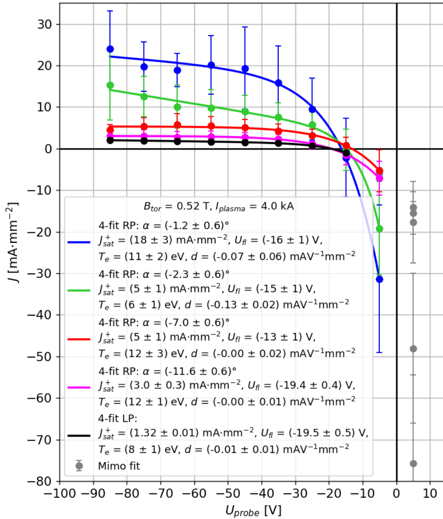
Obr. 3.23: Čtyři volt-ampérové charakteristiky získané metodou bin average z rail sondy (RP) pro různé úhly náklonu \alpha při magnetickém poli B_{tor} = 0,52 \text{ T} . Charakteristiky jsou doplněny o měření Langmuirovou sondou (LP, černá).
