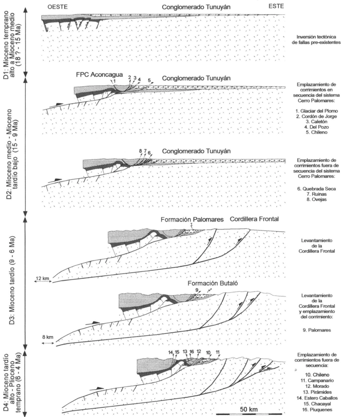
Figura 10: Esquema de evolución de la faja plegada y corrida del Aconcagua y de la Cordillera Frontal, donde se muestran los tiempos de emplazamiento de las distintas estructuras y su relación con los depósitos sinorogénicos.
