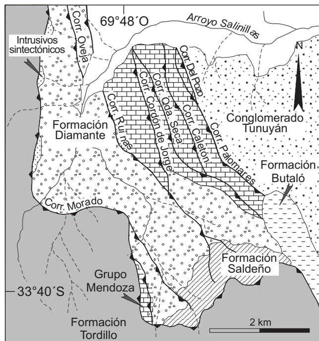
Figura 4: Mapa geológico de detalle del sistema de corrimientos Cerro Palomares del dominio estructural II. Se observan a los corrimientos en secuencia Cordón de Jorge, Caletón y del Pozo, y a los corrimientos fuera de secuencia Morado, Oveja, Ruinas, Quebrada Seca y Palomares. Nótese como algunas estructuras son cubiertas discordantemente por la Formación Butaló.
