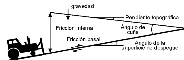
Figura 9: Esquema de cuña de Coulomb donde se muestran las variables que la modifican (Después de Davis et al. 1983).
