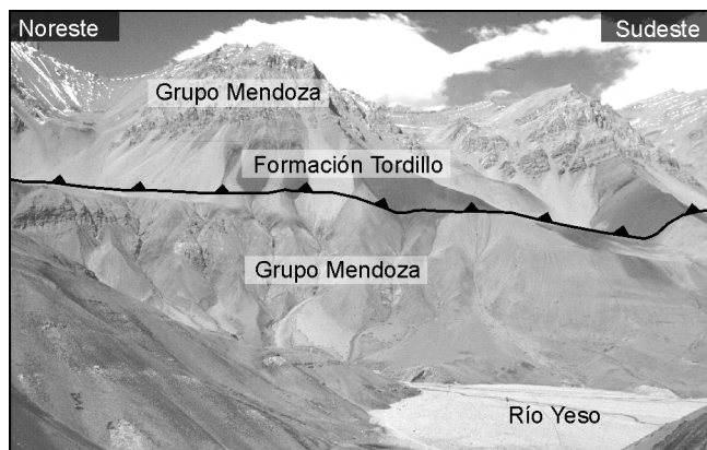
Figura 5: Fotografía mirando al sudeste desde el sector chileno, donde se observa al retrocorrimiento Glaciar del Plomo en el cordón del Límite.
