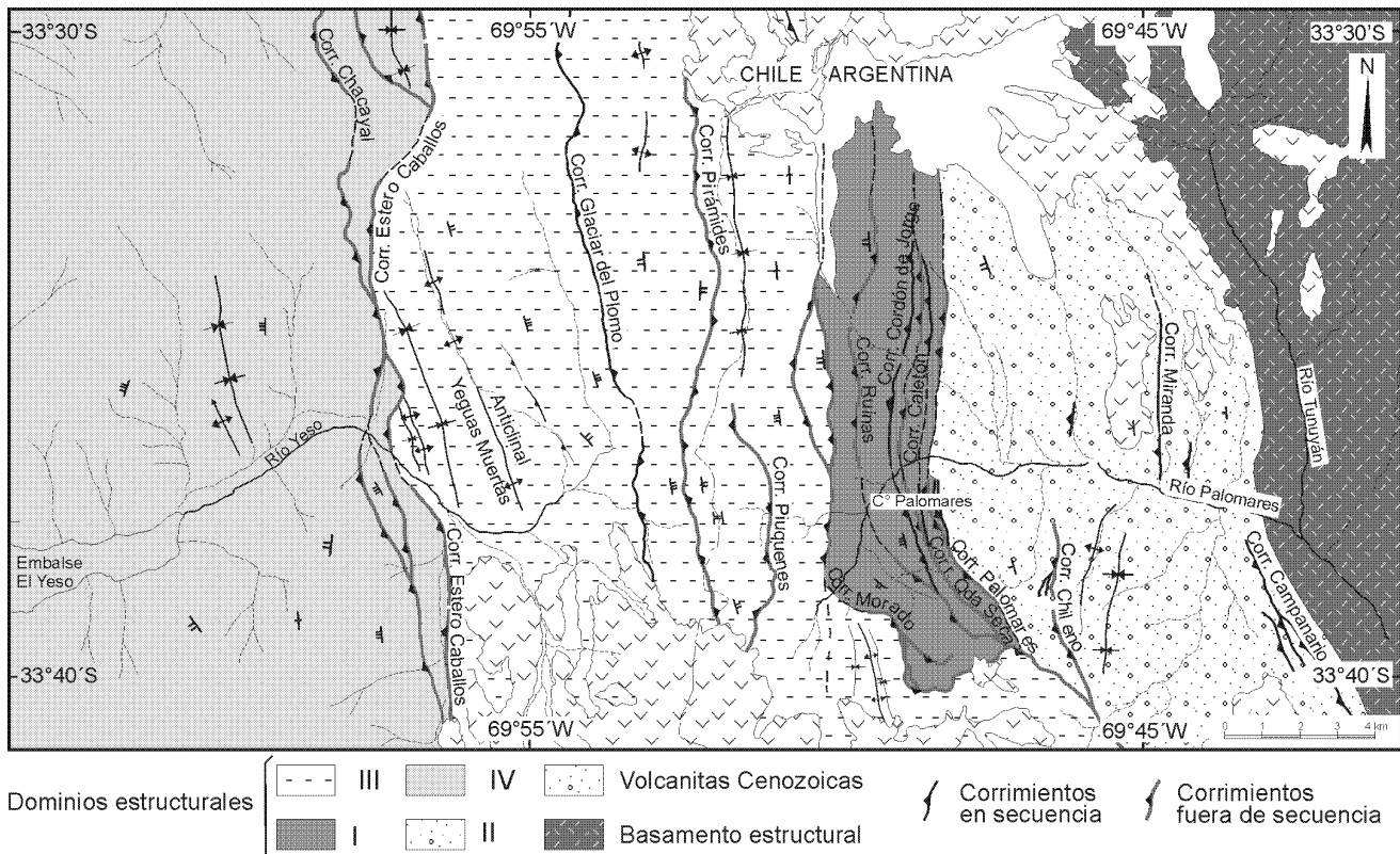
Figura 3: Mapa estructural simplificado, donde se muestran los cuatro dominios estructurales y se diferenciaron entre los corrimientos emplazados en secuencia de aquellos emplazados fuera de secuencia.
