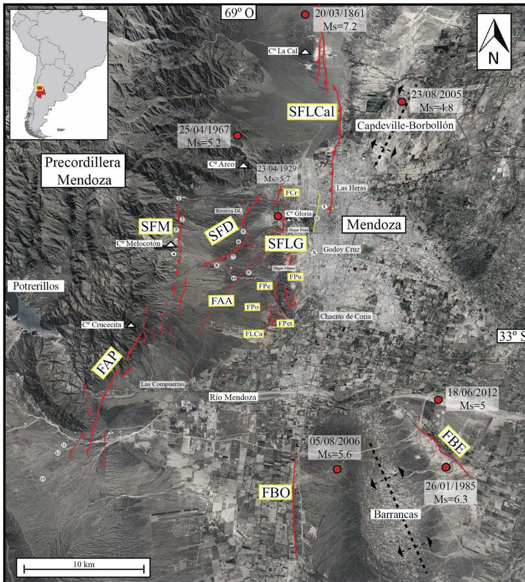
Figura 3 Imagen satelital 3D Landsat indicando trazas de las fallas con actividad cuaternaria del frente orogénico en el piedemonte mendocino: SFLCa: Sistema de fallas La Cal, SFLG: Sistema de fallas Cerro La Gloria, SFD: Sistema de fallas Divisadero Largo, SFM: Sistema de fallas Melocotón, FAA: Falla Agua de Las Avispas, FAP: Falla Agua de Pizarro, FBO: Falla Barrancas Oeste, y FBE: Falla Barrancas Este (modificado de Moreiras et al. , 2014; Toural-Dapoza y Moreiras, 2018; Toural-Dapoza et al. , 2019) y localización de epicentros de los principales sismos históricos (modificado de Schmidt et al. , 2011; Salomón et al. , 2013). Los diferentes puntos corresponden a los puestos: 1. San Isidro, 2. Chambón, 3. Las Trancas, 4. El Peral, 5. Colonia Papagayos, 6. Agua Batea, 7. Cienuguita, 8. Las Higuieritas, 9. Chilenos, 10. Agua Avispas, 11. La Saladita, 12. La Higuierita y 13. Jagüel; las calles de la ciudad de Mendoza mencionadas en el texto: I. Suipacha y II. Boulogne Sur Mer; mientras X corresponde al vecindario de Villa Marini en el departamento de Godoy Cruz.
