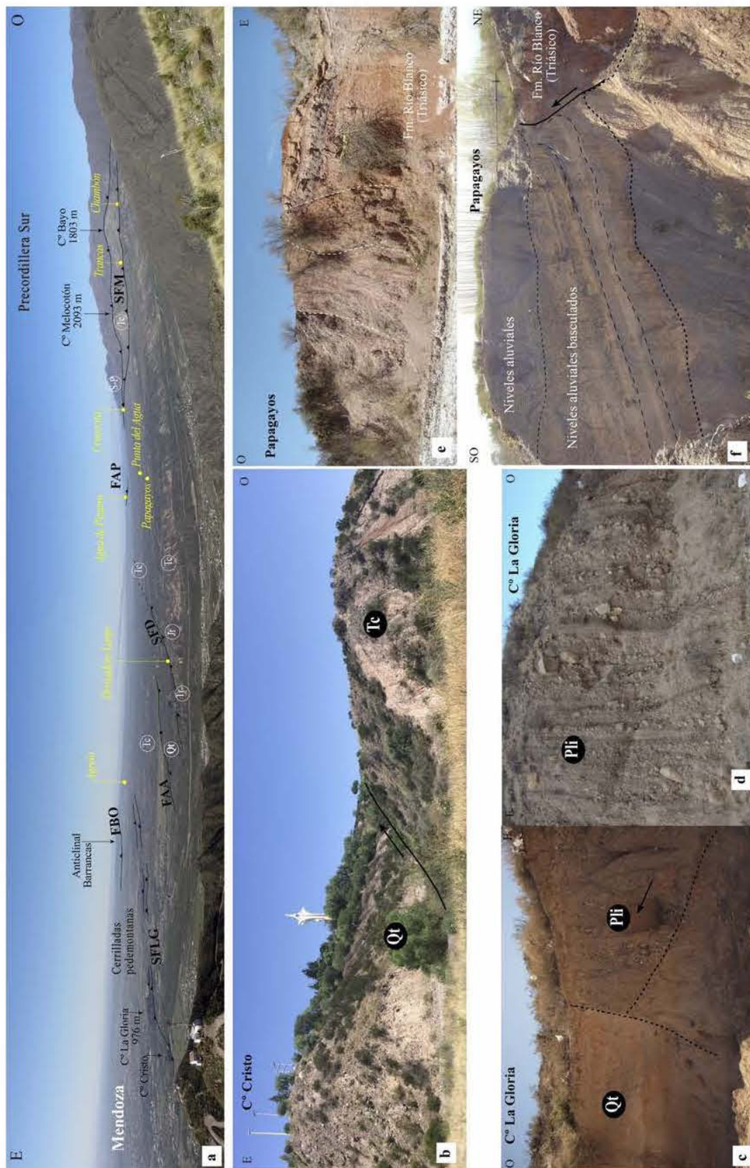
Figura 4 a. Foto Panorámica del piedemonte mendocino con el sistema de fallas cuaternarias: SFLG: Sistema de fallas La Gloria, FAA: Falla Agua de Las Avispas, SFD: Sistema de fallas Divisadero Largo, SFM: Sistema de fallas Melocotón, FAP: Falla Agua de Pizarro, y FBE: Falla Barrancas Este con las localidades típicas en color amarillo y edades de niveles: Qt: Cuaternario, Plio: Plioceno, Tc: Terciario, Jr: Jurásico y Tr: Triásico; b. Falla El Cristo afectando niveles aluviales cuaternarios y el neógeno; c. Falla Cerro de la Gloria A (N21°, Bz 32°E) en la ladera sur del cerro poniendo en contacto al Formación Mogotes con niveles lacustres de edad Pleistocena tardía (Bz12°O) y falla secundaria B (N33°, Bz 31°SE); d. Niveles de la Formación Mogotes verticalizados (N177, Bz 84°E) por la falla Cerro de La Gloria B ; e. niveles de la Formación Río Blanco deformados por la falla Divisadero Largo A en sector de Papagayos, y f. niveles de la Formación Río Blanco en contacto con niveles aluviales cuaternarios afectados por la falla Divisadero Largo Transcurrente (N126°,89°NO) que desplaza los segmentos A y B de la falla de Divisadero.
