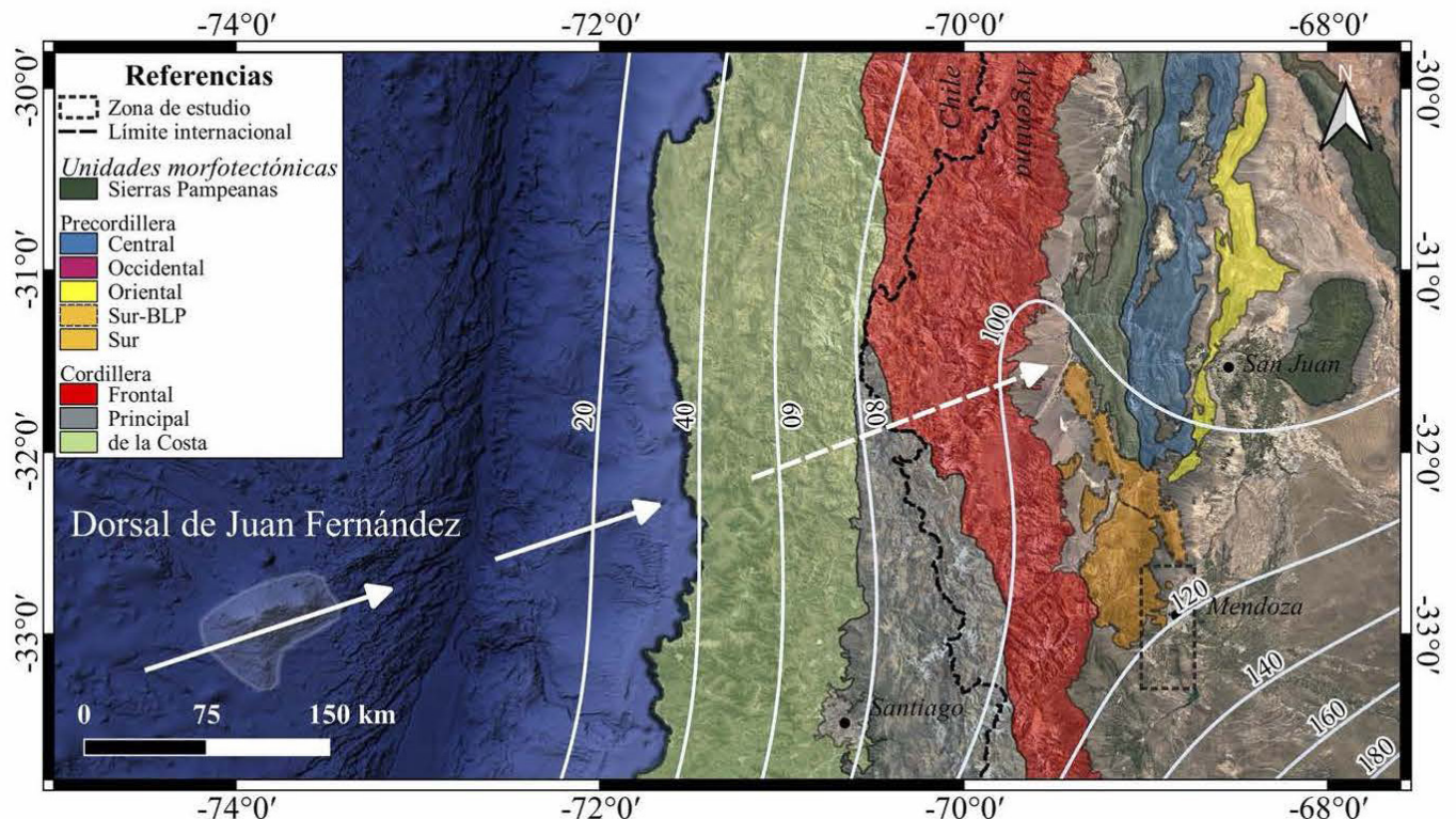
Figura 2 Mapa de ubicación de la zona de estudio mostrando las diferentes unidades morfoestructurales presentes en la región. El sentido y dirección de la dorsal de Juan Fernández son indicados por las flechas blancas. Los contornos de la geometría de la zona de Wadati-Benioff son mostrados con isolíneas en escala de color blanco-azul (superficial-profundo) y etiquetados en km según Hayes (2018).
