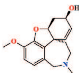
Galantamine
