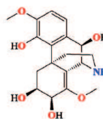
Tazopsine
