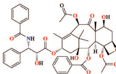
Paclitaxel (Taxol)
