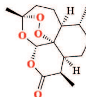
Artemisinin
