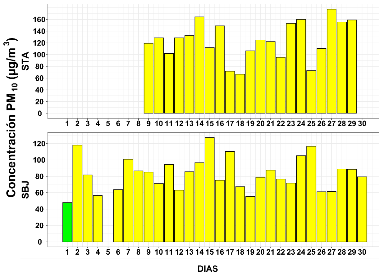
Figura N° 17. Estados de la Calidad del Aire para PM 10
