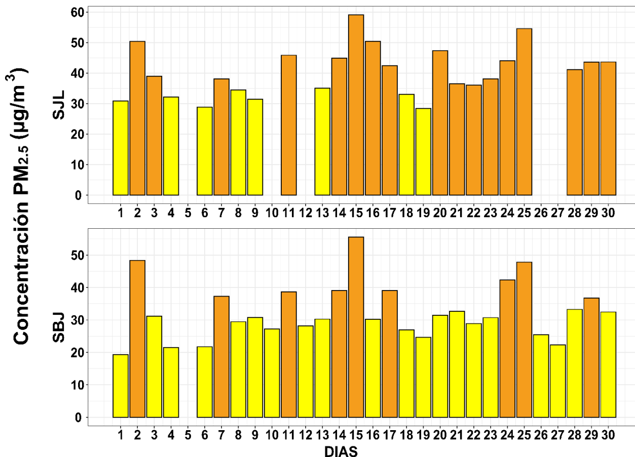
Figura N° 18. Estados de la Calidad del Aire para PM 2.5
