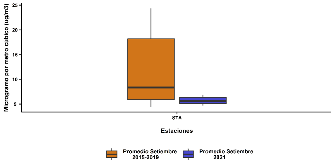
Figura N° 16. Comparativo entre las concentraciones históricas y las registradas durante el estado de emergencia para el O 3
