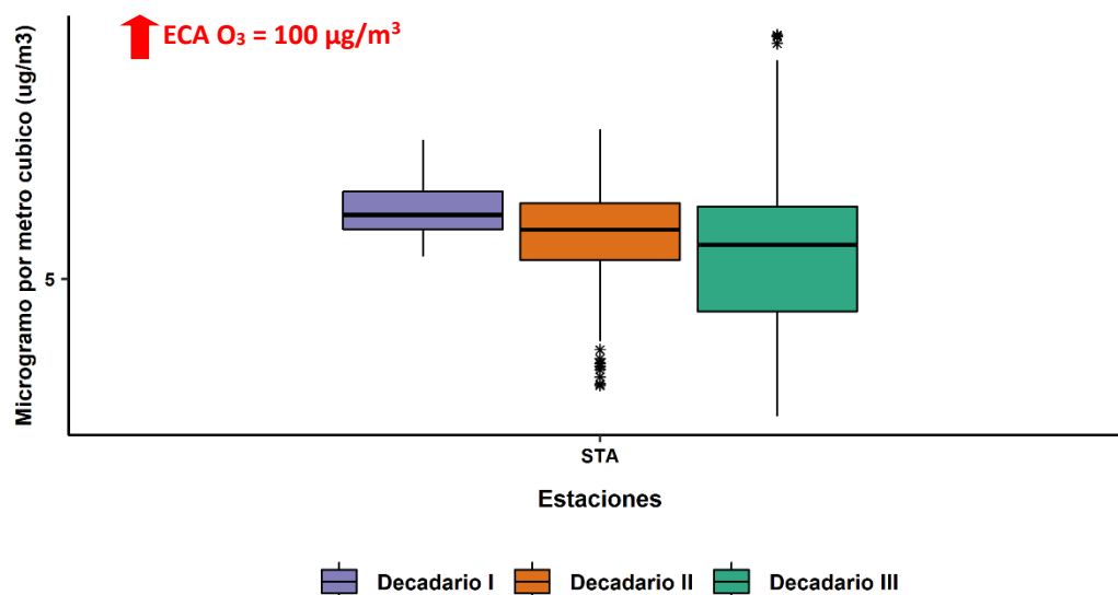
Figura N° 15. Variación horaria (promedio móvil de 8 horas) del O 3 (µg/m 3 ) en el AMLC.
