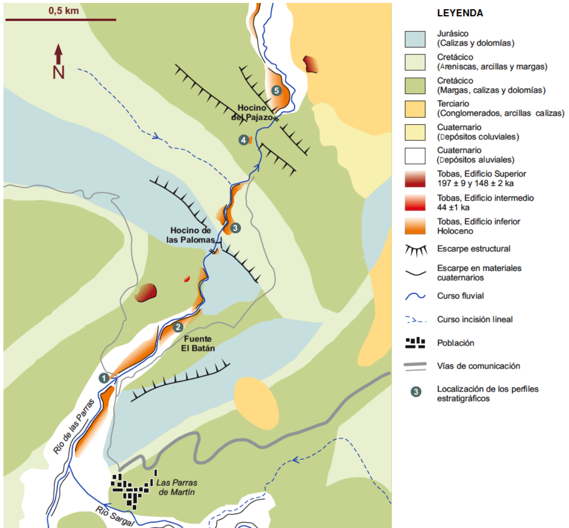
Figura 2. Esquema geológico y geomorfológico con la ubicación de los principales depósitos cuaternarios existentes en el valle del río Las Parras. Los depósitos holocenos 1 a 5 han sido analizados en Rico et al. (2013), mientras que las acumulaciones tobáceas de edad pleistocena se describen en Valero-Garcés et al. (2008). El depósito tobáceo del Nogal de El Batán se sitúa en el punto 2.
