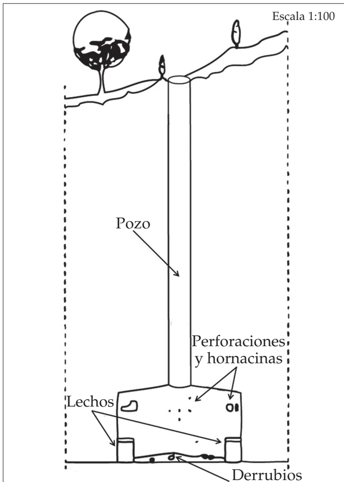
Figura 9 Sección transversal de la estancia I (elaboración propia según Monge y Jordán, 1993: 504)
