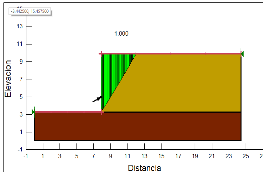
Figura 8. Factor de seguridad SLOPE/W del muro de contención de 6.00 m y talud 0°
