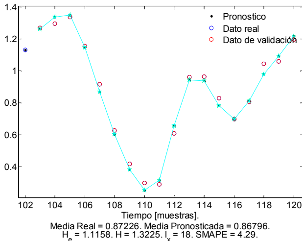
Fig. 6. Validación del pronóstico realizado sin decimación sobre la serie original.
