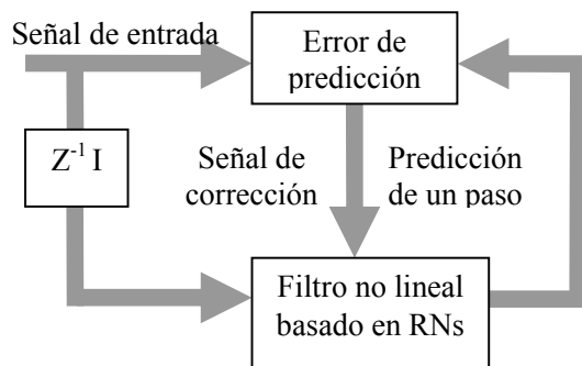
Fig. 3. Diagrama en bloques del sistema predictor.
