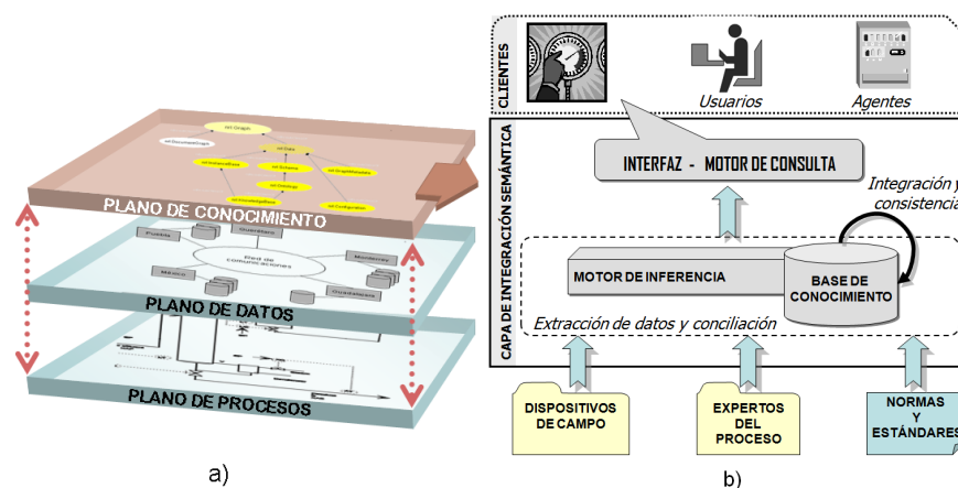
Fig. 1. Enfoque propuesto: a) Capa semántica en los SIPs b) Arquitectura de Integración
