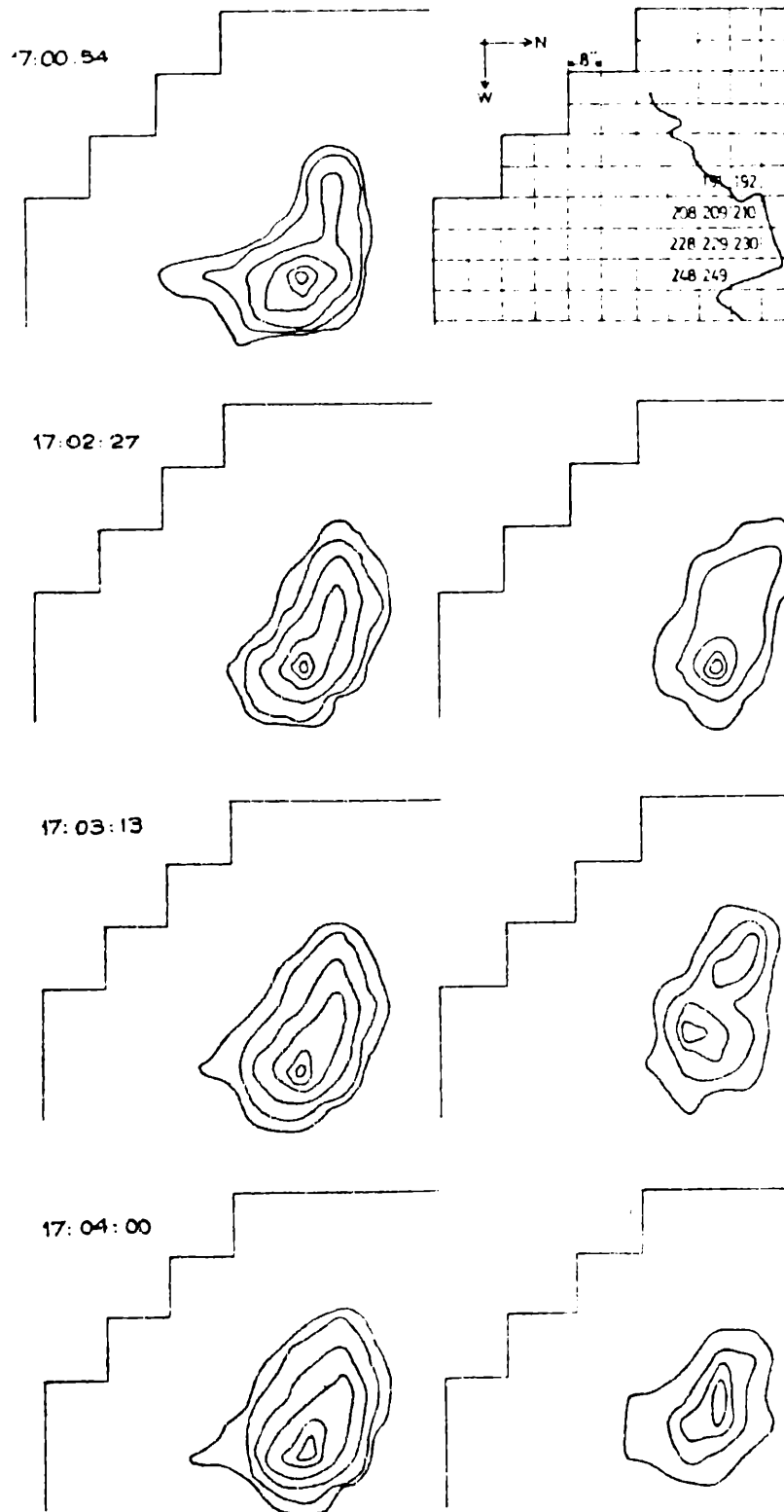
Figura 2: Contornos en rayos X blandos (3.5-5.5 keV) y duros (16-30 keV). El tiempo de integración es 22.5 segundos. Los niveles de los contornos son 90%, 75%, 50%, 25%, 10% y 5%. El nivel del 100% se indica en cuentas s^{-1} \text{ pixel}^{-1} en el extremo superior izquierdo de cada figura. En el cuadro superior derecho se ha superpuesto la línea neutra del campo magnético sobre los pixels del campo fino.
