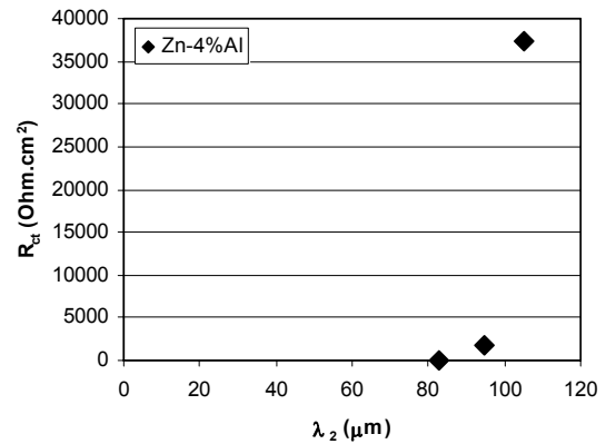
Figura 10. Correlación de la R_{ct} con el \lambda_2 .
