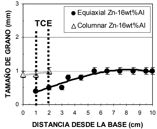
Figura 4. Tamaño de grano versus distancia desde la base de la muestra. (a) ZA4. (b) ZA16.
