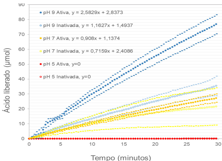
Figura 1. Ácidos graxos liberados quando polpas maceradas de dendê ativas (círculos cheios) e inativadas (círculos vazios) foram utilizadas como substratos. Os ensaios foram realizados em valores de pH 5 (gráficos vermelhos), pH 7 (gráficos amarelos) e pH 9 (gráficos azuis) em meios reacionais emulsificados. Os traços nas respectivas cores dos círculos indicam os valores da média \pm desvio padrão.
