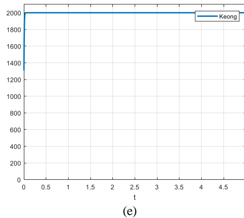
Gambar 2. Simulasi Numerik Model Transmisi Penyakit Schistosomiasis : (a) Dinamika Sub-populasi Manusia Rentan, (b) Dinamika Sub-populasi Manusia Terinfeksi Schistosomiasis , (c) Dinamika Sub-populasi Larva Miracidia , (d) Dinamika Sub-populasi Cercaria , dan (e) Dinamika Populasi Keong O.h. lindoensis
