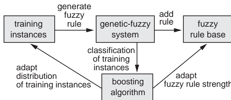
Figure 3. Modelo basado en algoritmos evolutivos (Hoffmann, Baesens, Mues, Gestel, & Vanthienen, 2007)
