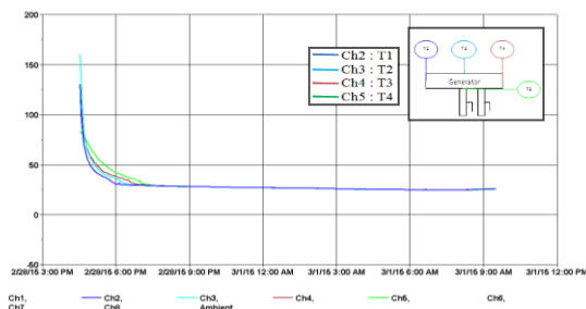
Gambar 4.11 Grafik Temperatur vs Waktu Adsorpsi Alat Penguji Adsorpsi (amonia) tanpa fin
