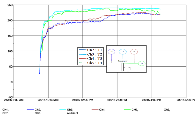
Gambar 4.2 Grafik Temperatur vs Waktu Pemvakuman Alat Penguji Adsorpsi (amonia) menggunakan Fin
