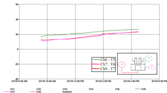
Gambar 4.18 Grafik Temperatur vs Waktu Desorpsi Gelas Ukur Refrigerant (amonia)
