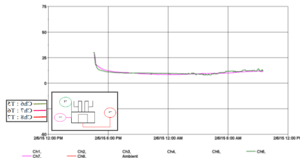
Gambar 4.9 Grafik Temperatur vs Waktu Adsorpsi Gelas Ukur Refrigerant (amonia)
