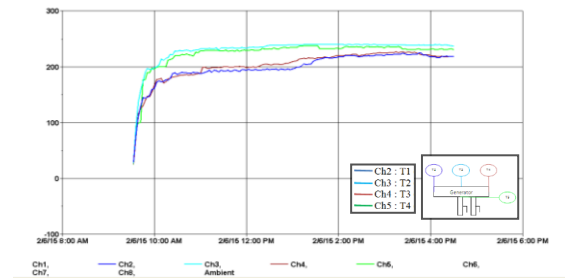
Gambar 4.14 Grafik Temperatur vs Waktu Desorpsi Alat Penguji Adsorpsi (amonia) menggunakan fin
