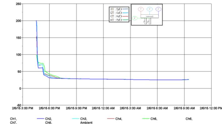
Gambar 4.8 Grafik Temperatur vs Waktu Adsorpsi Alat Penguji Adsorpsi (amonia) menggunakan fin
