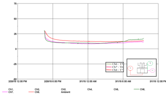
Gambar 4.12 Grafik Temperatur vs Waktu Adsorpsi Gelas Ukur Refrigerant (amonia)
