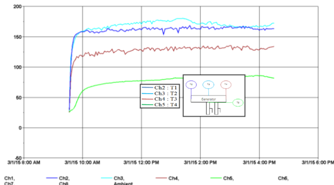
Gambar 4.17 Grafik Temperatur vs Waktu Desorpsi Alat Penguji Adsorpsi (amonia) tanpa menggunakan fin
