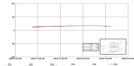
Gambar 4.15 Grafik Temperatur vs Waktu Desorpsi Gelas Ukur Refrigerant (amonia)
