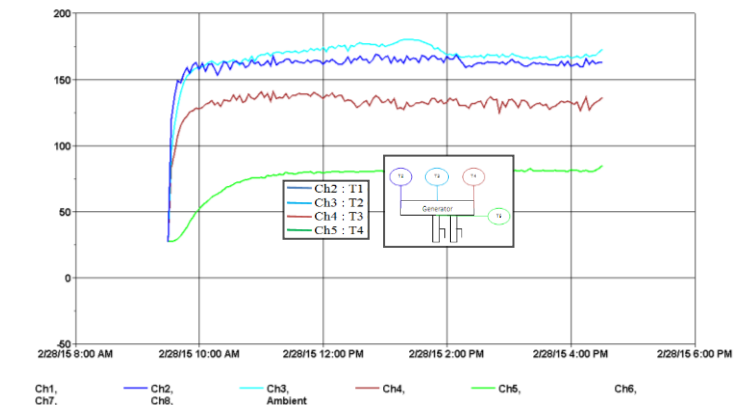
Gambar 4.5 Grafik Temperatur vs Waktu Pemvakuman Alat Penguji Adsorpsi (Amonia) tanpa fin
