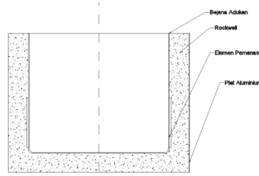
Gambar 9 Konstruksi Insulation Material pada Elemen Pemanas
