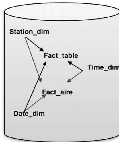
Fig. 2. ESTRUCTURA DE LA BODEGA DE DATOS
