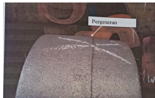
Gambar 3.3 Cacat pergeseran
