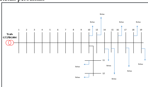
Gambar 8 Single Line Diagram Jurusan A Setelah Perbaikan
