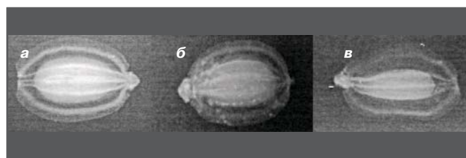
Рис. 3. Рентгенографические изображения семян укропа пахучего: а – с выполненным зародышем; б – с грибным повреждением; в – с невыполненным зародышем
