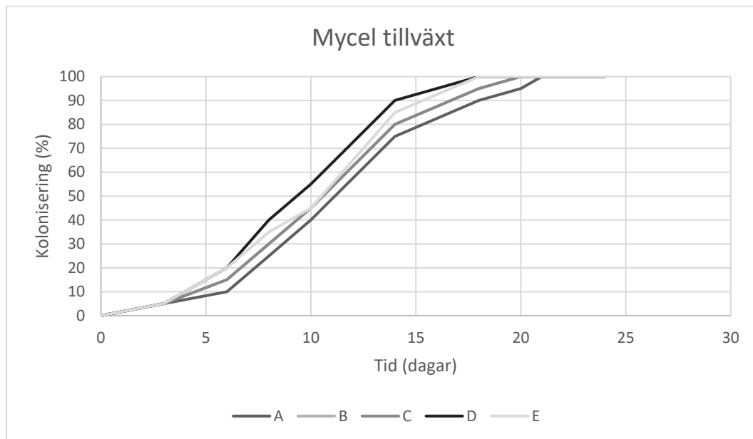
Figur 6. Mycel tillväxt
