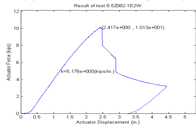
(d) t=0.082 in. ( M_{test}/M_y=0.94 )
