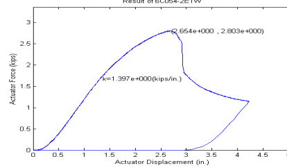
(d) h=6 in. ( M_{test}/M_y=1.06 )
