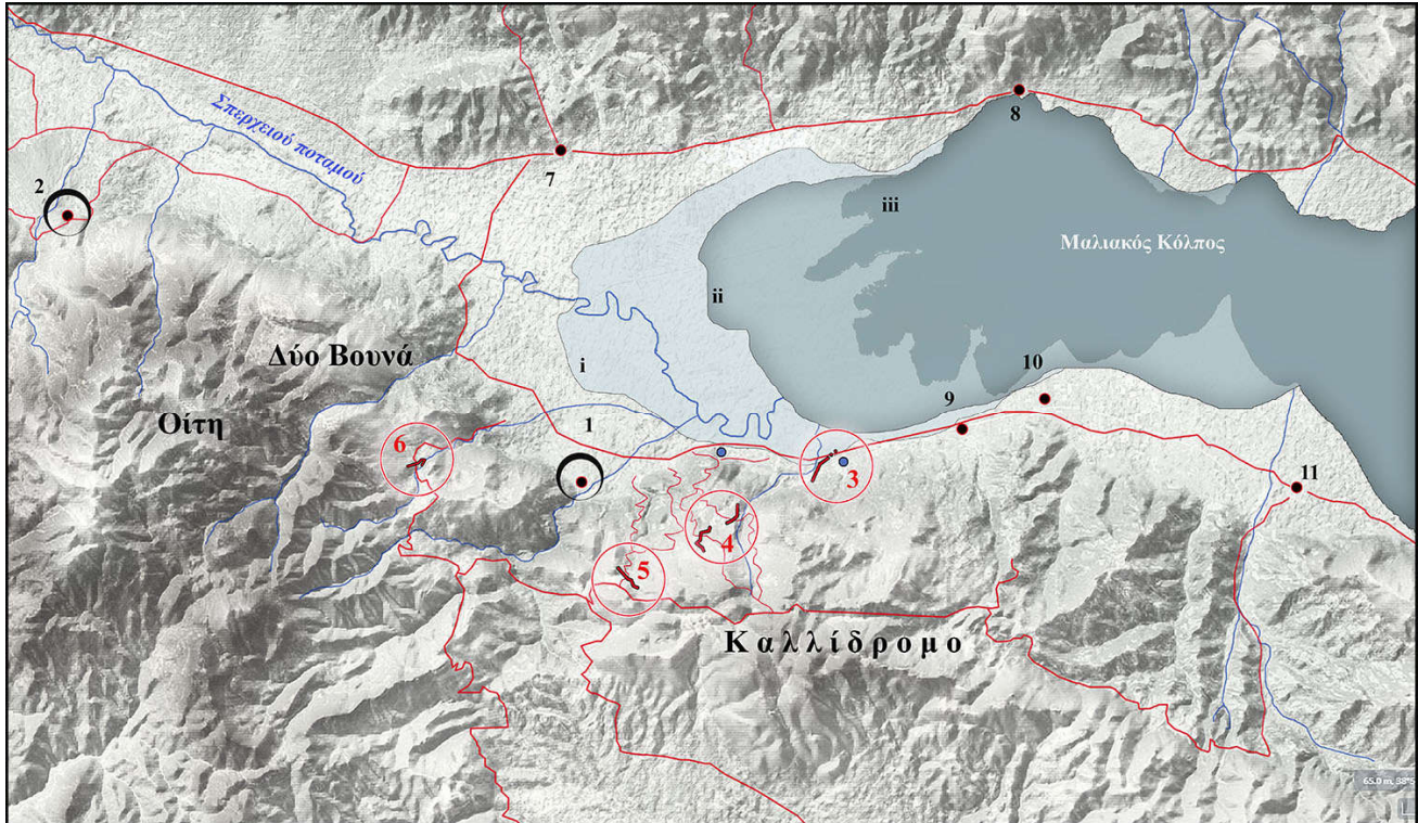
Слика 14 - Општа диспозиција запречних бедема који су чинили Јустинијанов систем клаустре у подручју Термопила на седлима планина Калидромос и Дуо Вуна. Два града која су посебно добила сопствене бедеме од Јустинијана јесу (1) Хераклеја Трахинија и (2) Хипате (Υπάτη) који су бранили прилазе речним долинама у свом залеђу. Систем није чинила једна линијска баријера него неколико стратешки постављених бедема по превојима на које је избијало више планинских путева од којих је према Прокопију нарочито опасан по јужне провинције био пут преко Дуо Вуне у залеђу Хераклеје. Данас познат под именом Дема теснац (κλεισούρας), пролаз је затворен изградњом археолошки евидентираних тврђава о којој је и Прокопије писао – Миропол (Μυροπόλεις). На главном преградном зиду (διјатихизми) између планине Калидромос и морске обале (i. линија обале 480. старе ере, ii. оквирна контура обале у VI веку и iii. данашња обала Малијског залива - Μαλιακός Κόλπος) и северно од топлих извора, археолошки су установљени главни бедем са кружном кулом и протеихизмом избаченој 5m ка северу, као и доста опеке што је можда индиција да је тај бедемски систем једини био изведен у опус микстум техници. Клаустре: 3. Термопили, 4-5. Седла на планини Калидромо, 6. Тврђава Миропол. Остала насеља: 7. Ламија, 8. Фалара, 9. Алпенос, 10. Никеја. 11. Скарфија. (Maskau, Procopius' De Aedificiis and the Topography of Thermopylae, 241-255; Kraft et al., The Pass at Thermopylae, 181-198; Cherf, The Dhema Pass, 144)
