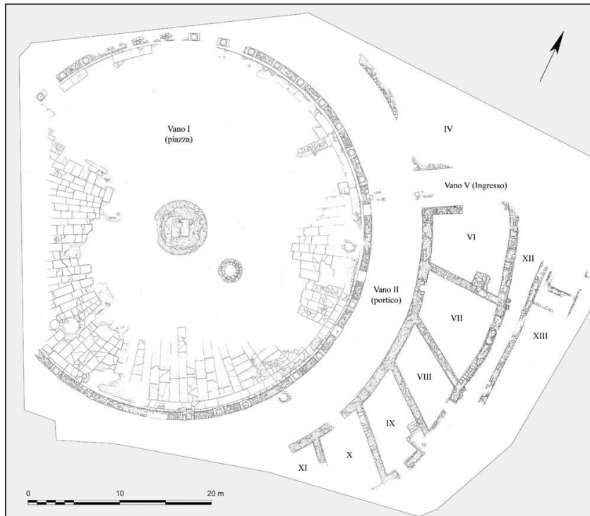
Слика 11 - План велике пјачете мацелума у Дирахијуму са приказом просторија радњи у спољном прстену око кружне стое са неубичајеним габаритним поделама у односу на круг пјаче. ( Baronio, Il cosiddetto macellum-forum di Durazzo, Fig.5 )
