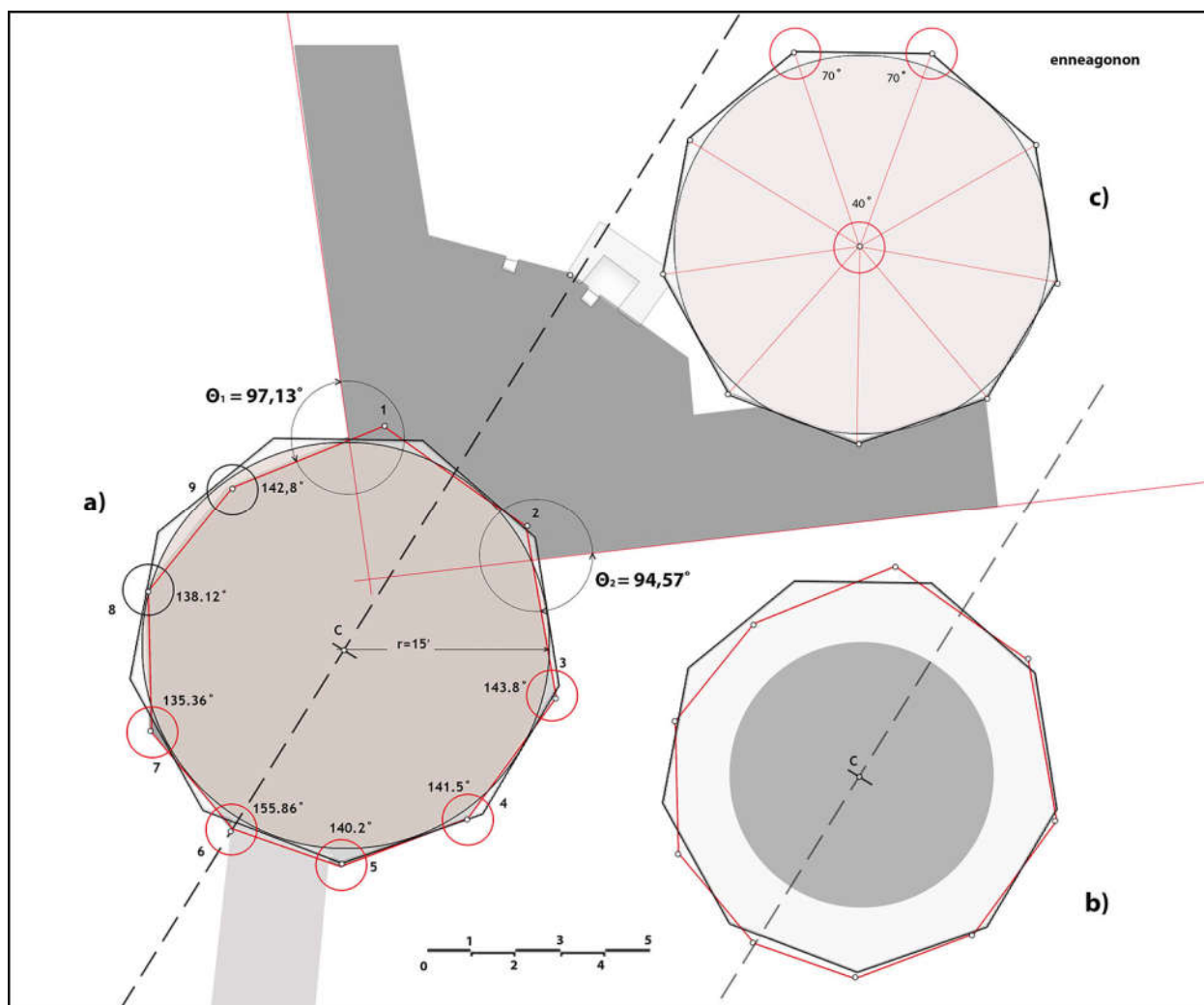
Слика 34 - Прелиминарна геометријска анализа деветоугаоне контуре основе Водене куле Горњег града са установљењем одступања од углова који важе за правилни деветоугао где су углови по правилу при центру полигона 40^\circ а по периметру 140^\circ степени.
