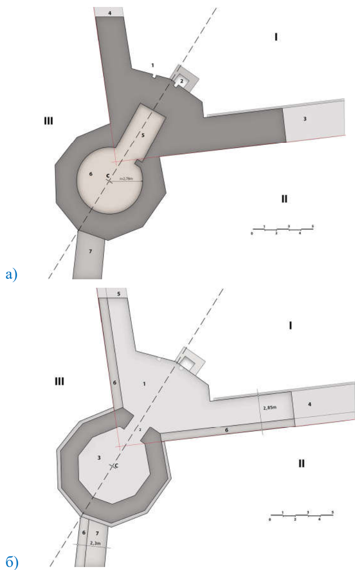
Слика 33 - План полигоналне (деветоугаоне) основе субструкције Водене куле на југозападном углу бедема Горњег града. Геометријска поставка приказа прати изведено стање које је претрпело прилагођавања волумена куле топографским условима па је симетрија грађевине унеколико нарушена. Основне реперне осе јесу симетрална подужна линија и приближно ортогонални угао два бедемска платна Горњег града. а) Основа базе куле са дводелним резервоаром и прикључцима на бедеме где је доводна траса аквадукта ишла дуж западног зида Доњег града. б) Основа спрата са предлогом полигоналне контуре зидова у унутрашњости који прате полигоналну базу куле. Унутрашњост је могла да буде изведена и на кружној основи.
