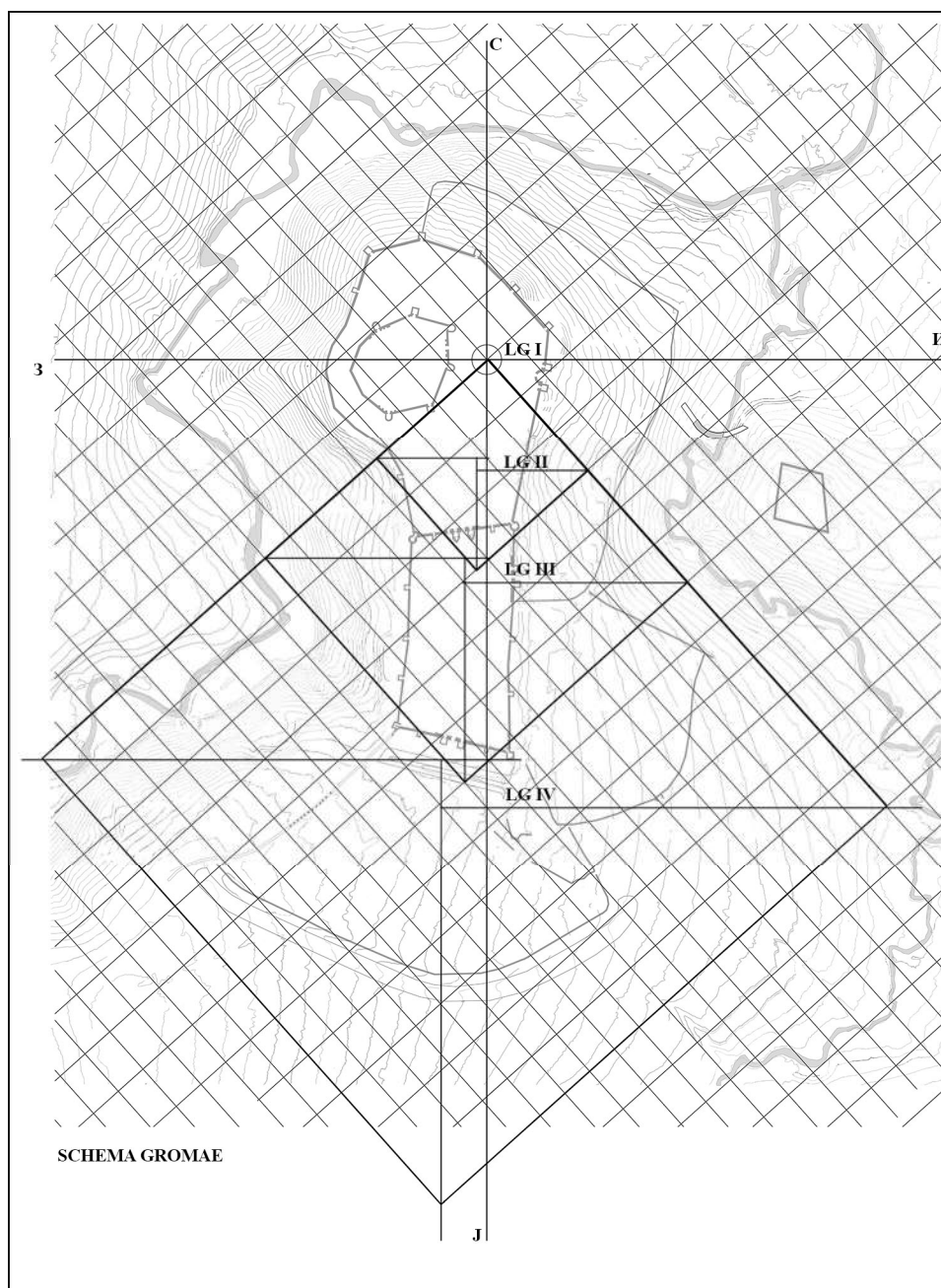
Слика 28 - SCHEMA GROMAE , геометријска процедура за распоређивање геодетских станица - грбма у оквиру хексадецималне премерне мреже методом ad quadratum . Схема приказује геометријски принцип уз помоћ којег се гробе лако могу поставити на терен користећи кардиналне правце. Наравно, велики квадрати са удаљеним теменима се нису трасирали на терену али су зато 'модусни' квадрати са гробма у свом средишту свакако били обележени јер су осим места гробе, давали могућност контроле исправности визирања кардиналних праваца, нарочито правца север-југ са почетком из средишта форума.
