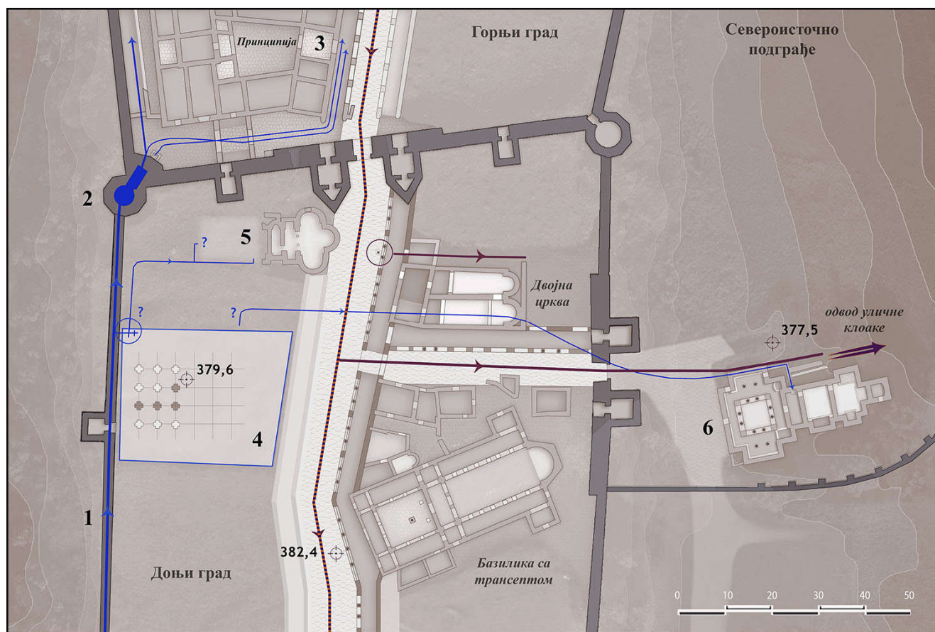
Слика 25 - План хидрауличног чворишта у Доњем граду са евидентираним трасама оловних цеви за развод свеже воде у Горњем граду и претпостављеним прикључцима других снабдевачких разводних линија чија места извода из резервоара цистерне нису истражени. Укупно посматрано, развођење тијаће односно свеже воде посебним системом из резервоара Водене куле за Горњи град и складиштење великих залиха допремљене воде у пространи резервоар Велике цистерне говори о устаљеној и простудираној методи прорачуна и пројектовања инсталације не само према потребним количинама воде на бази дневне потрошње него и о умећу стриктног или рутинског спровођења режима контролисане потрошње. План је исцртан преко подлоге ортофотограметријског снимка Царичиног града, док су три висинске коте преузете из Петровић, О водоводу Царичиног града, Сл. 3. 1. Траса аквадукта, 2. Водена кула Горњег града, 3. Развод ка форуму Горњег града, 4. Велика цистерна, 5. Мало купатило – balnae , 6. Велике терме.
