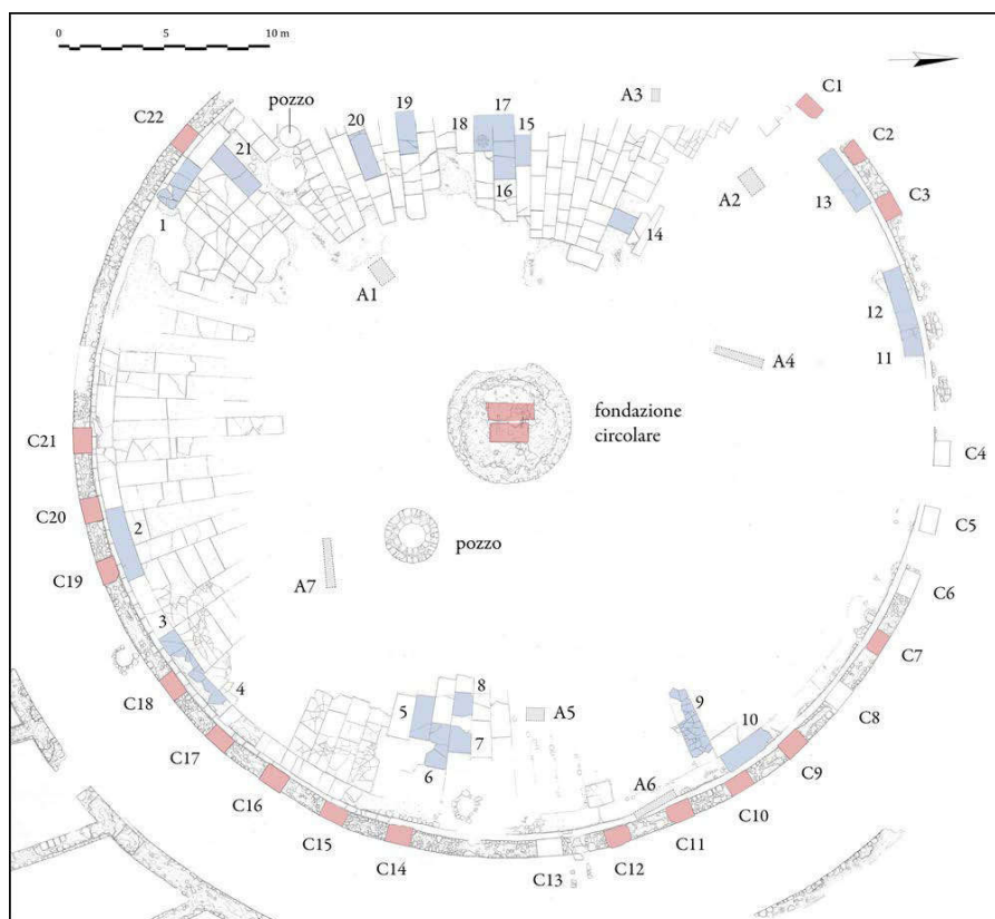
Слика 12 - План велике пјацете мацелума у Дирахијуму са уцртаним стилобатом и плинтама база стубова кружне стое (црвено) и плавом бојом означеним мермерним плочама са епиграфским урезима и симболима. ( Baronio, Il cosiddetto macellum-forum di Durazzo, Fig.12 )
