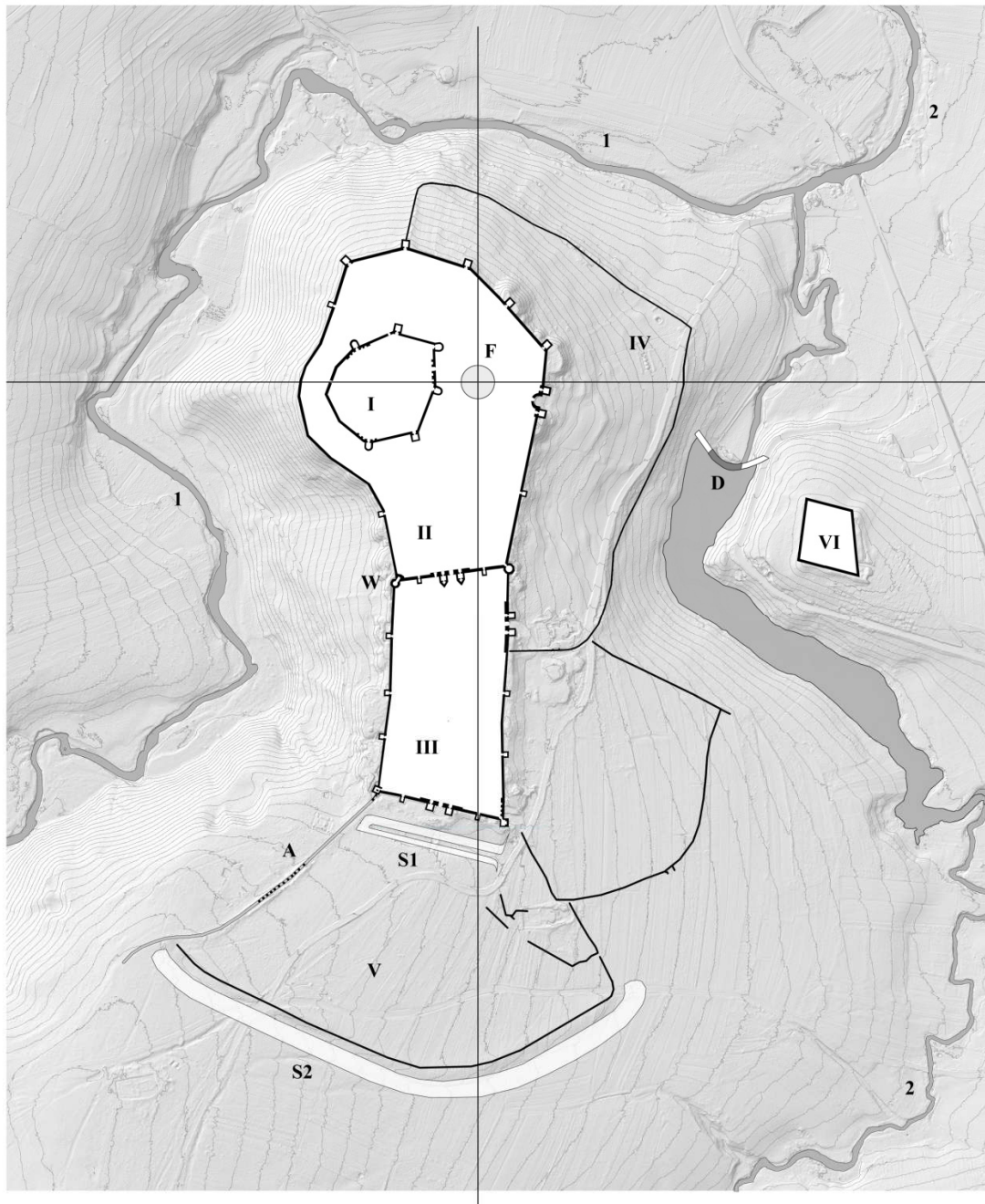
Слика 27 - Општа диспозиција фортификацијских радова на Царичином граду (Јустинијани Прими). Фортификација: I. Акропољ, II. Горњи град, III. Доњи град, IV. Североисточно подграђе, V. валум (vallum), VI. квадрибургијум на брегу Свети Илија. Референтне грађевине: F – форум (forum), A – аквадукт, W – Водена кула, D – брана на Царичинској реци, S1, S2 – градски ровови, фосе (fossa). Топографски маркери: 1. Река Свињарица, 2. Царичинска река. Куле северно од Источне капије Горњег града нису истражене али су позната њихова места.
