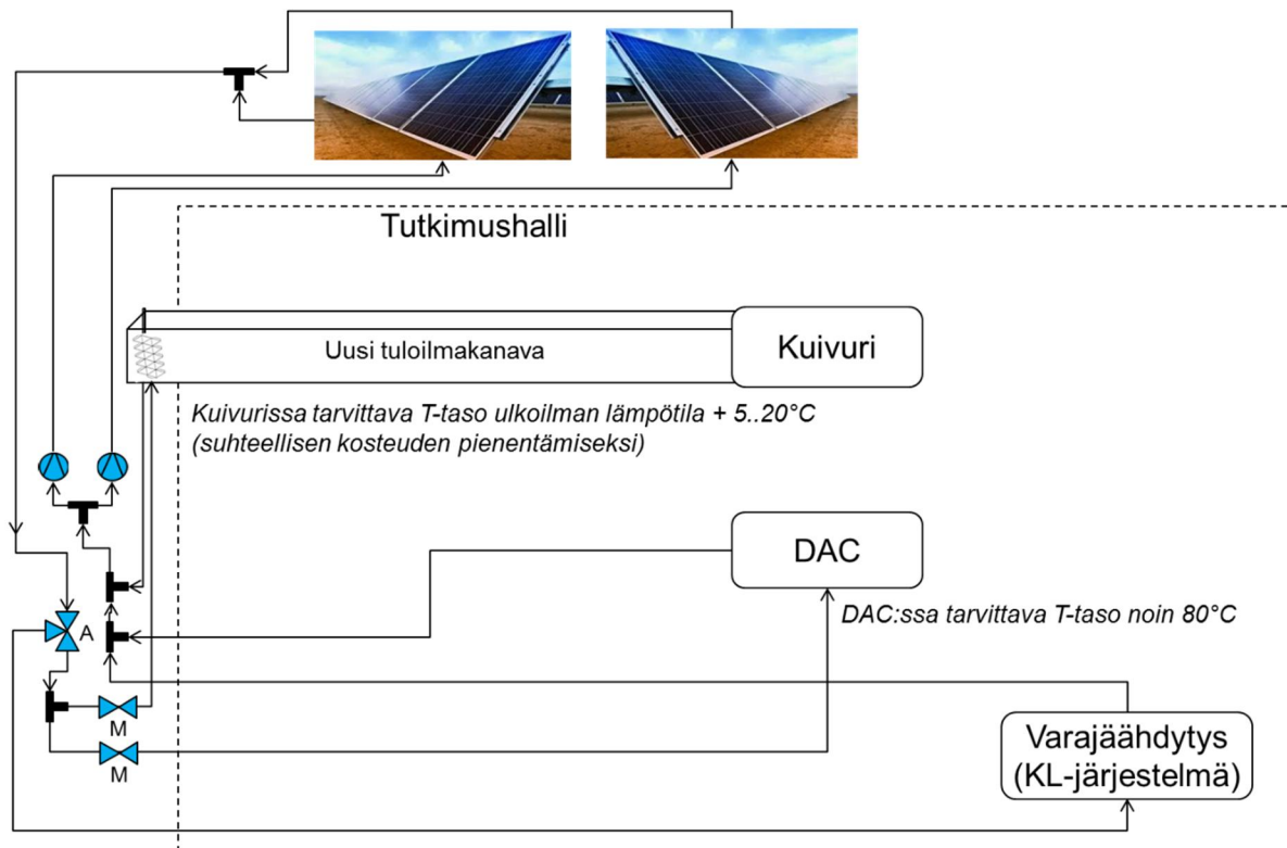
Kuva 16. Aurinkojärjestelmän periaatekuva
