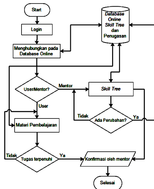
Gambar 1. Model Pengembangan Pemrograman Produk.
