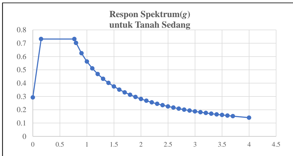
Gambar 4. Respon Spektrum (Sumber : puskim.pu.go.id )
