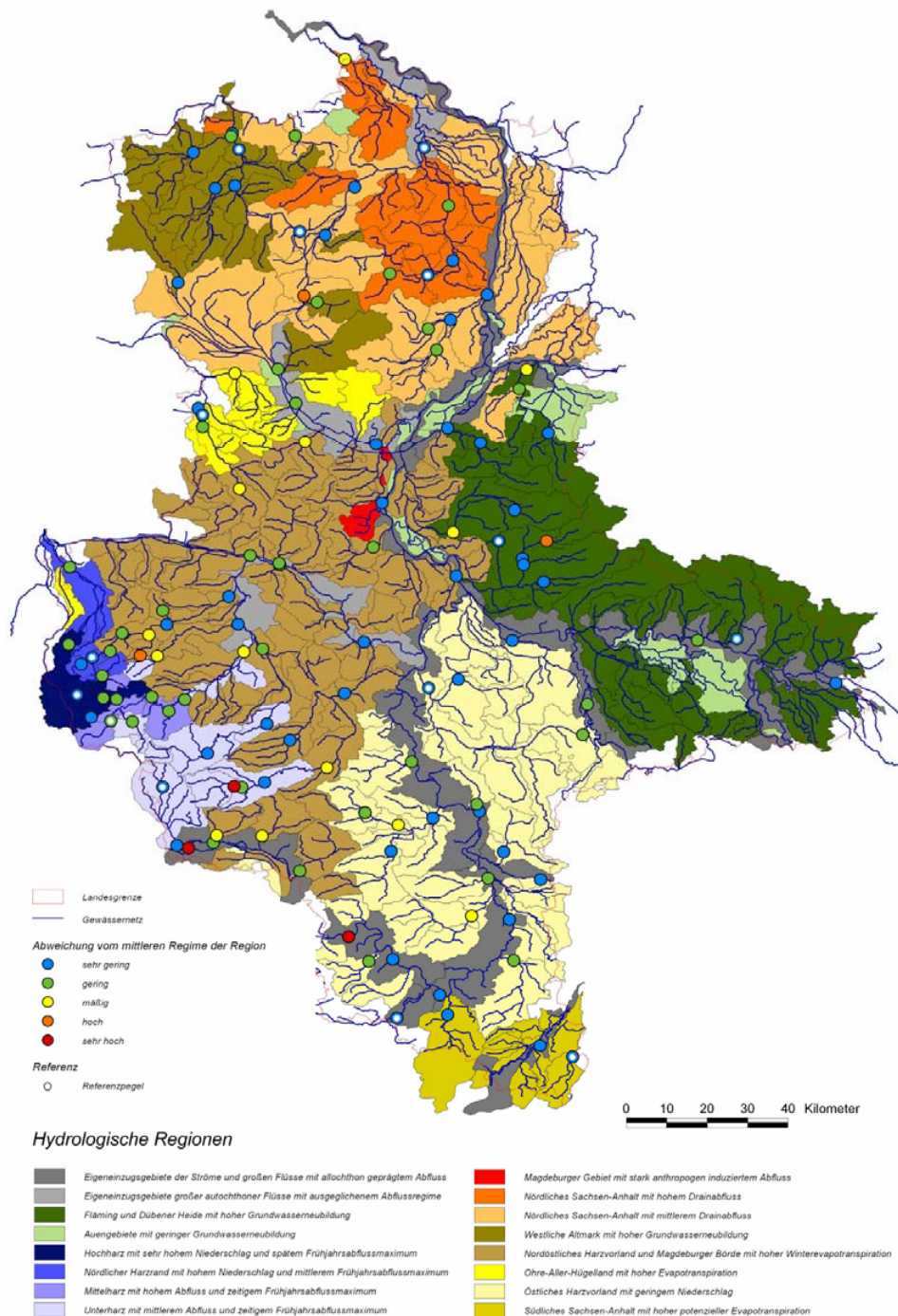
Abb. 4: Hydrologische Regionen und Abweichungen der Pegelregime vom mittleren Regime. Fig. 4: Hydrological regions and deviations of the gauged flow regimes from the mean regime.
