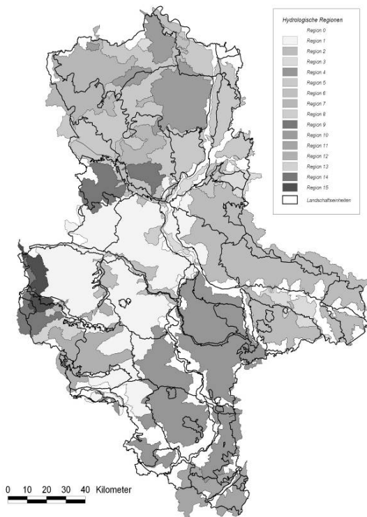
Abb. 5: Lagevergleich Hydrologische Regionen und Landschaftseinheiten von Sachsen-Anhalt (Quelle: LAU 2000).
