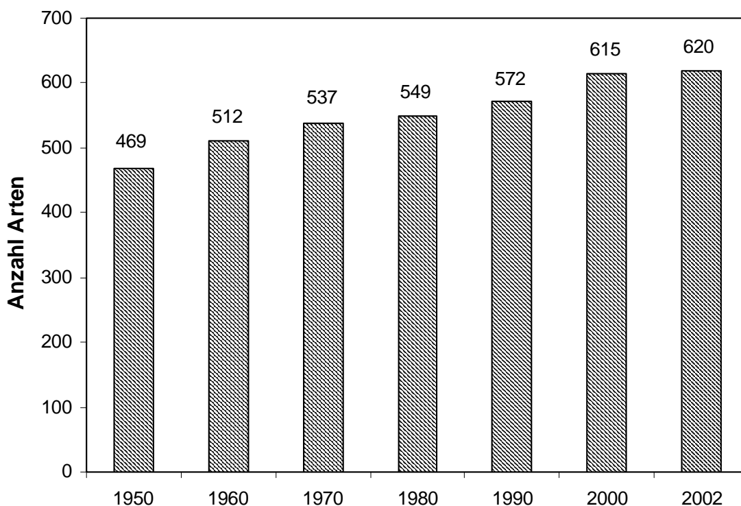
Abb. 1: Zikadenartnachweise in Deutschland seit 1950. Neuzugänge wurden gewertet zum Zeitpunkt des ersten Nachweises bzw. nach dem Erscheinen von Revisionen und Neubeschreibungen. — Numbers of Auchenorrhyncha species known from Germany since 1950. Additional records were counted at the time of the first record or after the publication of taxonomic revisions and original descriptions, respectively.
