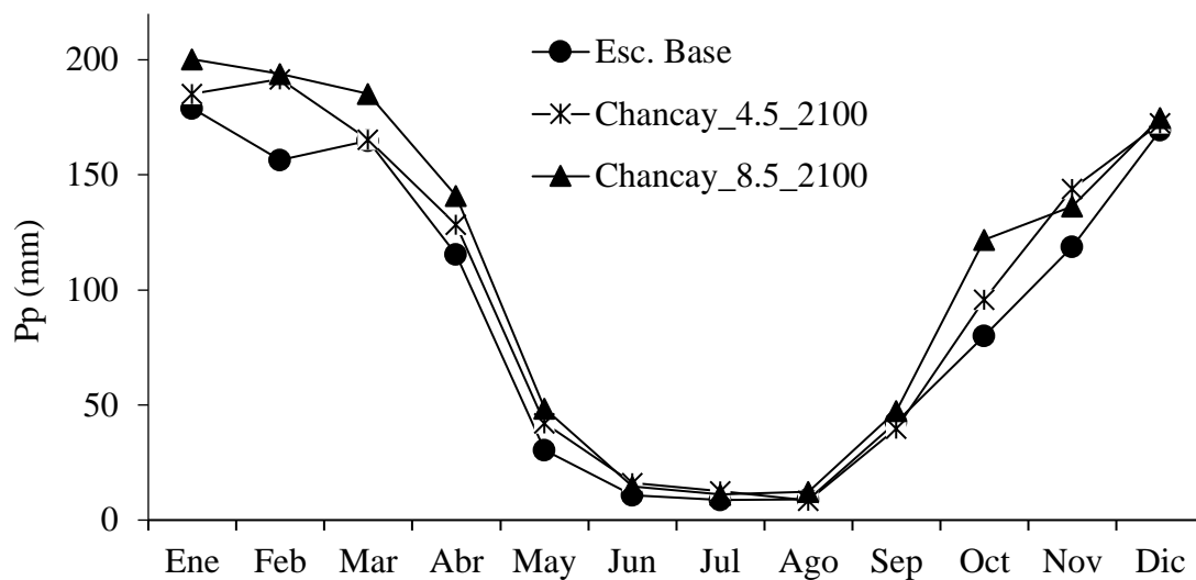
Figura 10: Precipitación media observada y modelo CNRM-ESM 2-1 estación Chancay.
