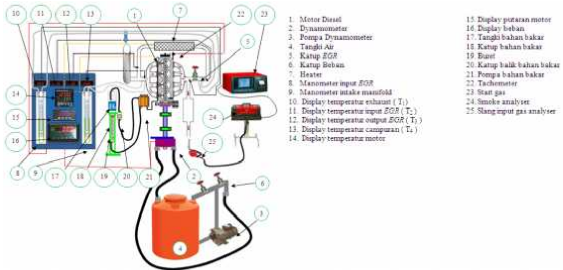
Gambar 3.2. Setup eksperimen
