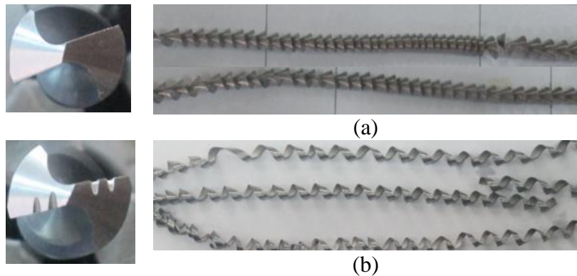
Gambar 2. Chip morfologi pada pengeboran dengan twist drill tanpa splitting nick (a) dan chip morfologi pada pengeboran dengan twist drill yang diberikan splitting nick (b)
