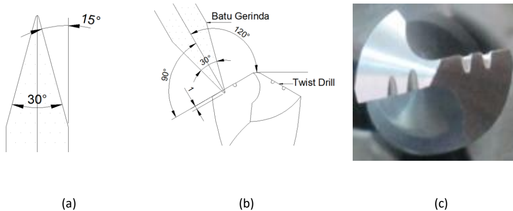
Gambar 1. (a) Dimensi batu gerinda (b) Desain penggerindaan Mata bor twist drill dengan splitting nicks (c) Mata bor dengan splitting nicks hasil penggerindaan dengan mesin tool grinding
