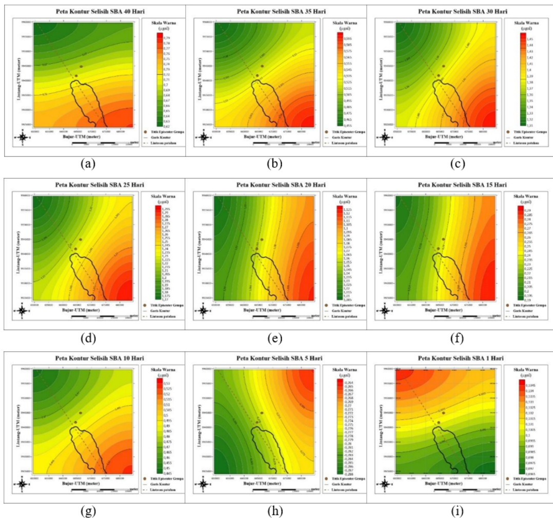
Gambar 3 Polarisasi nilai SBA pada episenter (a) 40 hari, (b) 35 hari, (c) 30 hari, (d) 25 hari, (e) 20 hari, (f) 15 hari, (g) 10 hari, (h) 5 hari, (i) 1 hari sebelum dengan sesudah terjadinya gempa
