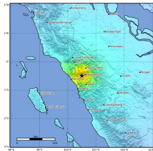
Gambar 2 Peta gempa 6 Maret 2007 magnitudo 6,4 dengan titik episenter ditandai dengan simbol bintang
