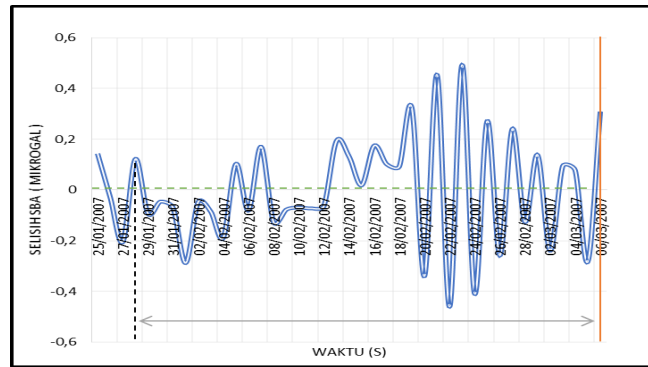
Gambar 5 Grafik selisih harian SBA di episenter gempa 6 Maret 2007 magnitudo 6,4
