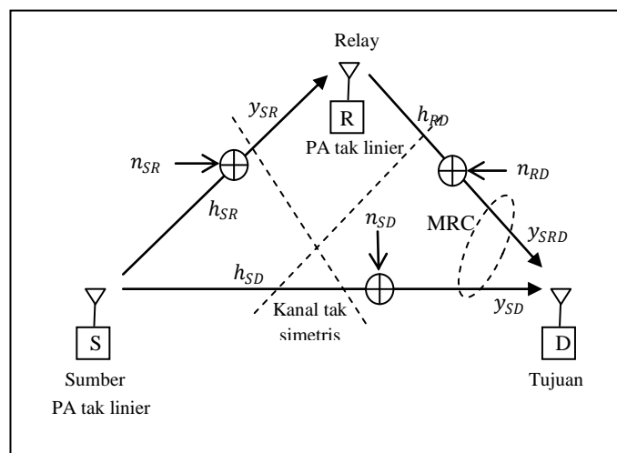
Gambar 1. Diagram jaringan komunikasi kooperatif dengan kanal tak simetris.
