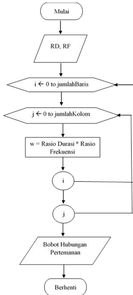
Gambar 3. 4 Tahapan Perhitungan Bobot Hubungan Pertemanan
