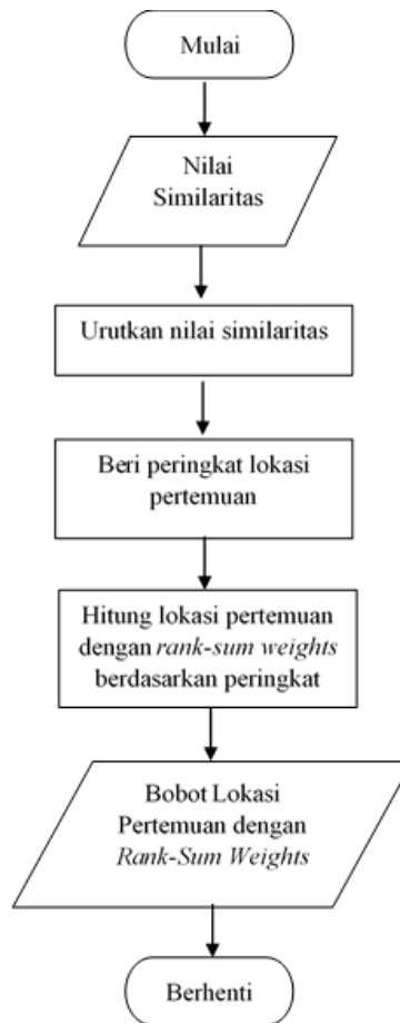
Gambar 3. 8 Tahap Perhitungan Lokasi Pertemuan ( Rank-Sum Weights )
