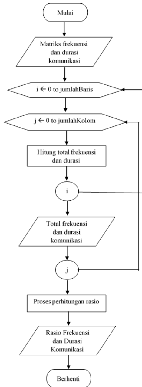
Gambar 3. 3 Tahapan Perhitungan Rasio Frekuensi Komunikasi
