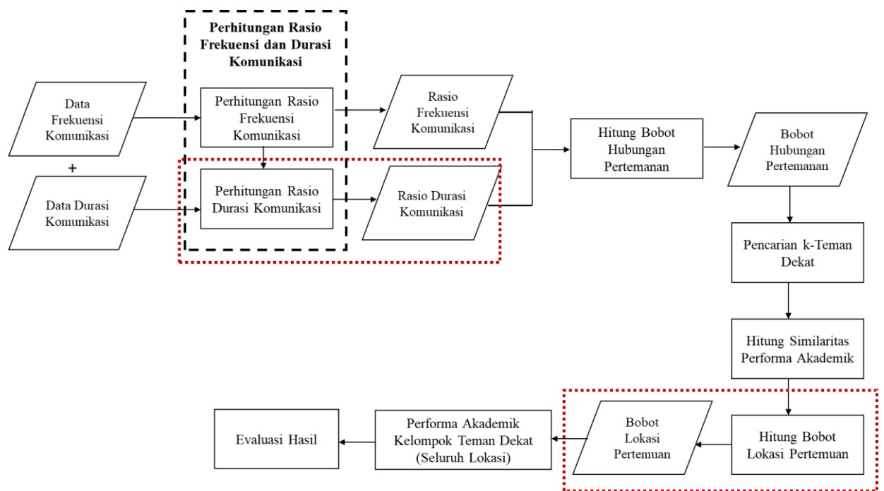
Gambar 3. 2 Diagram Alir Usulan Metode Penelitian
