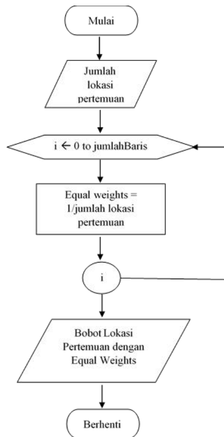
Gambar 3. 5 Tahap Perhitungan Lokasi Pertemuan ( Equal Weights )
