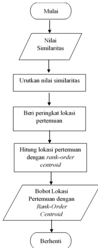
Gambar 3. 7 Tahap Perhitungan Bobot Lokasi Pertemuan ( Rank-Order Centroid )
