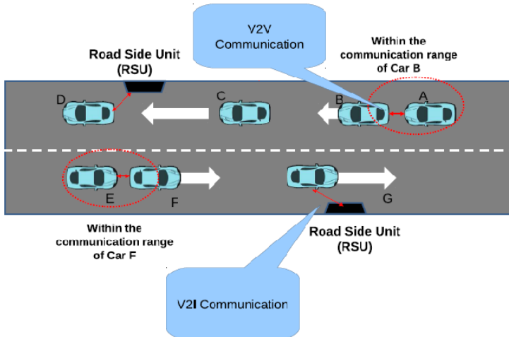
Gambar 2.1 Ilustrasi VANET
